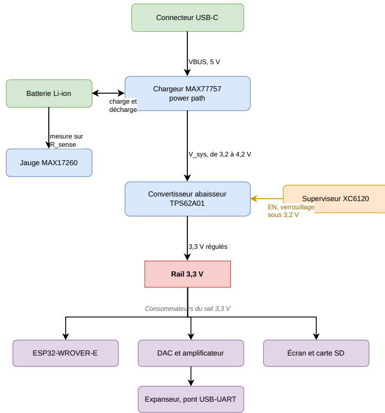
Figure 4.1 – Arbre d'alimentation, de l'entrée USB au rail logique
