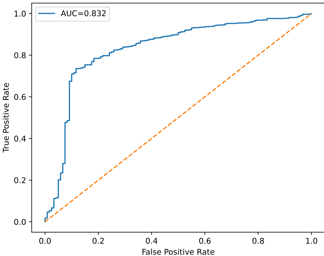
ROC — autoencoder
