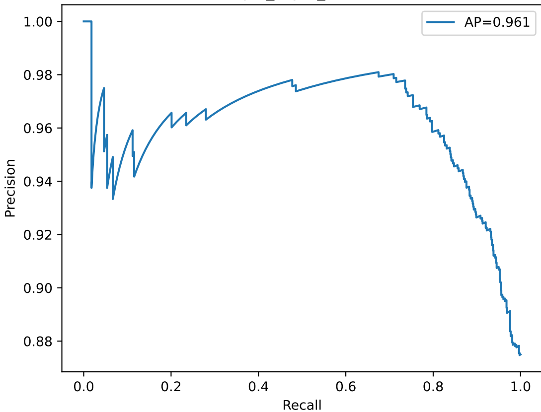
PR — tfqkd_asym_autoencoder
