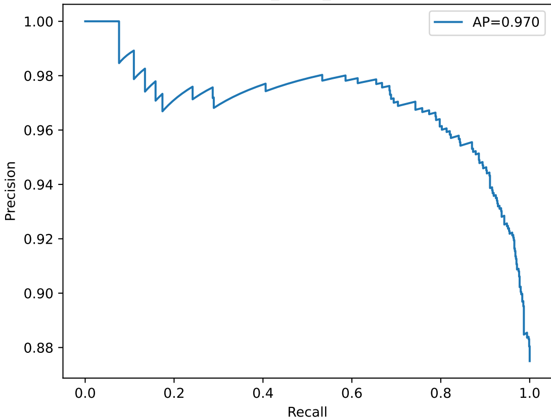
PR — tfqkd_clean_autoencoder
