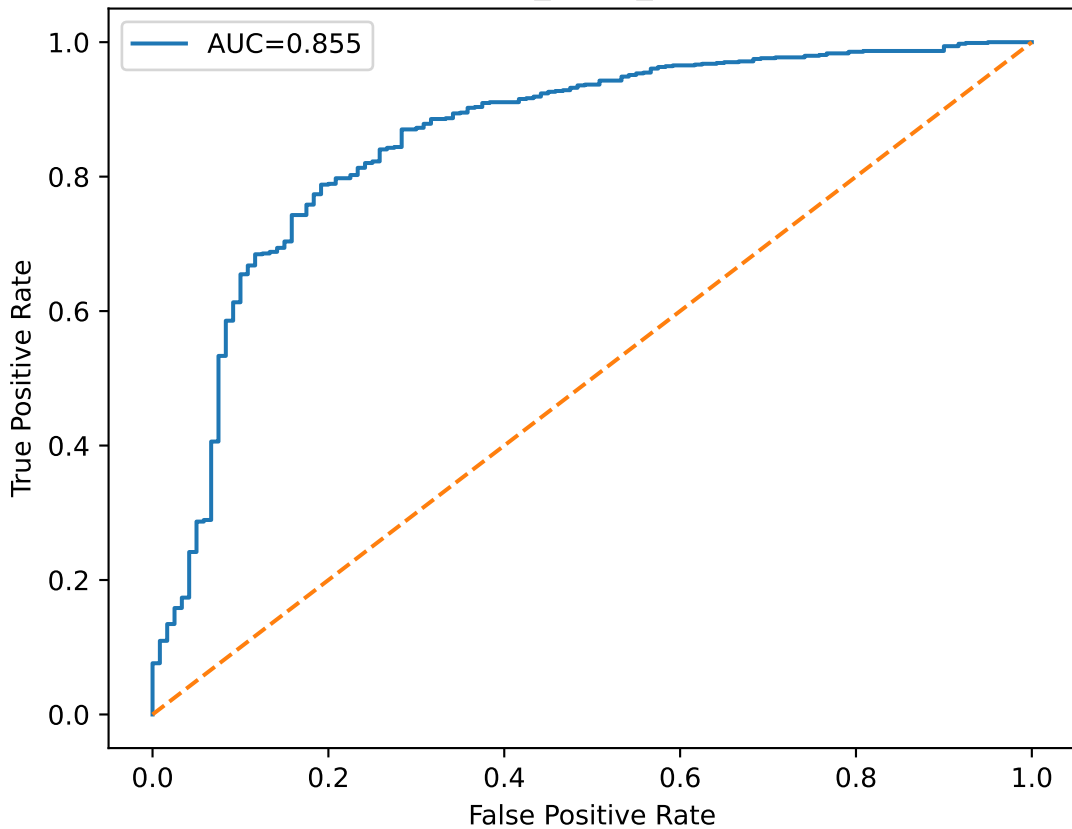
ROC — tfqkd_clean_autoencoder
