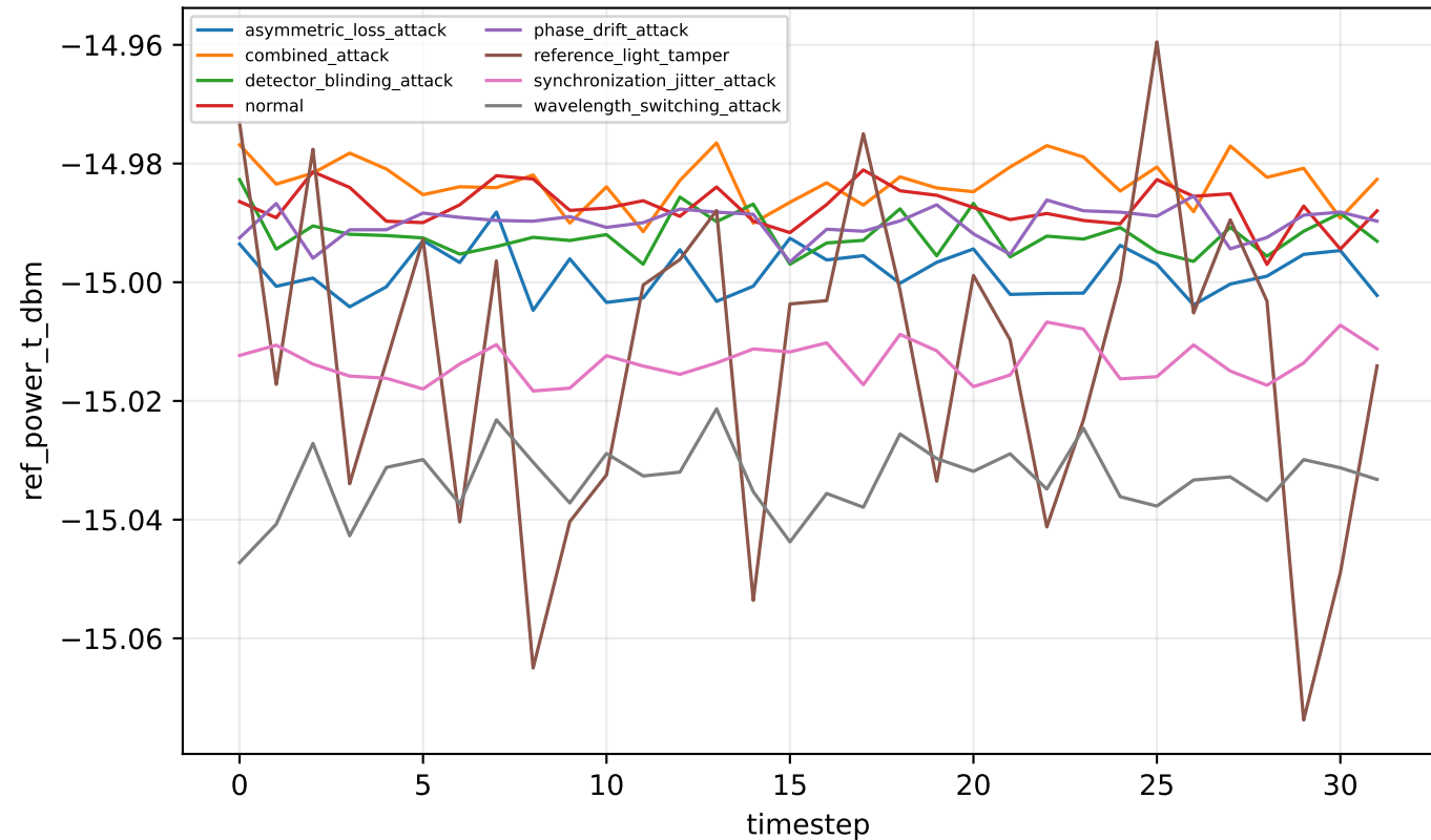
tfqkd_drift — ref_power_t_dbm
