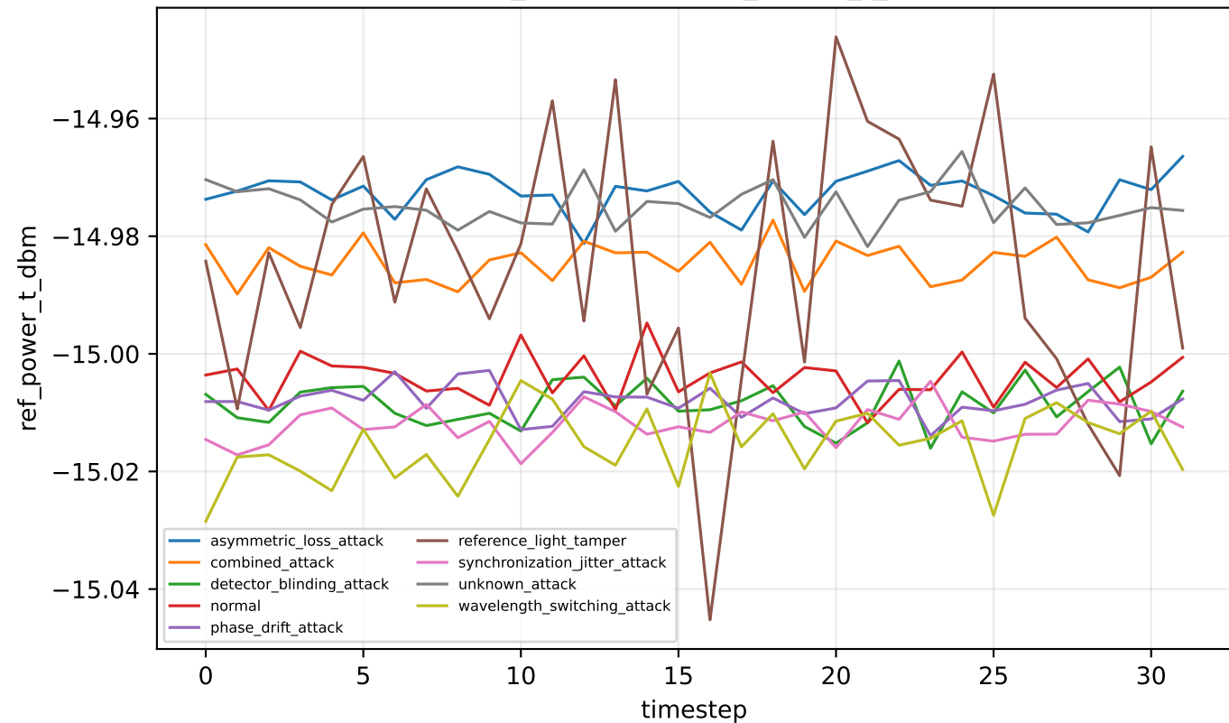
tfqkd_unknown — ref_power_t_dbm
