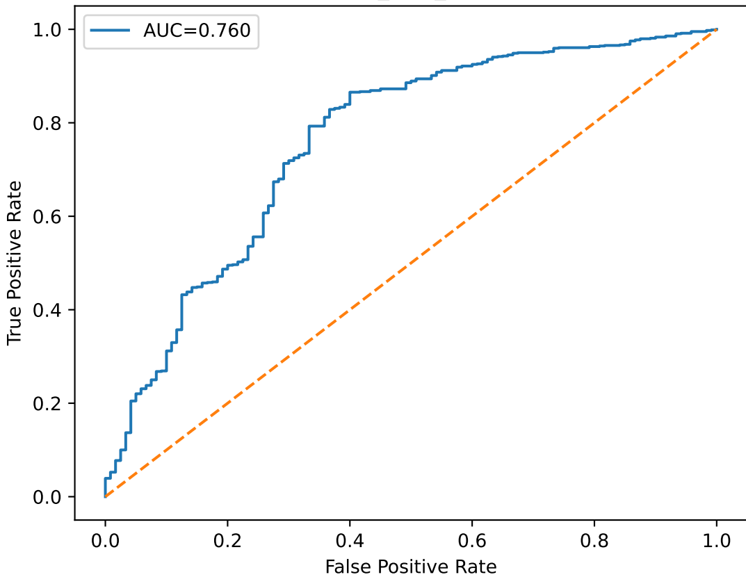
ROC — tfqkd_drift_autoencoder
