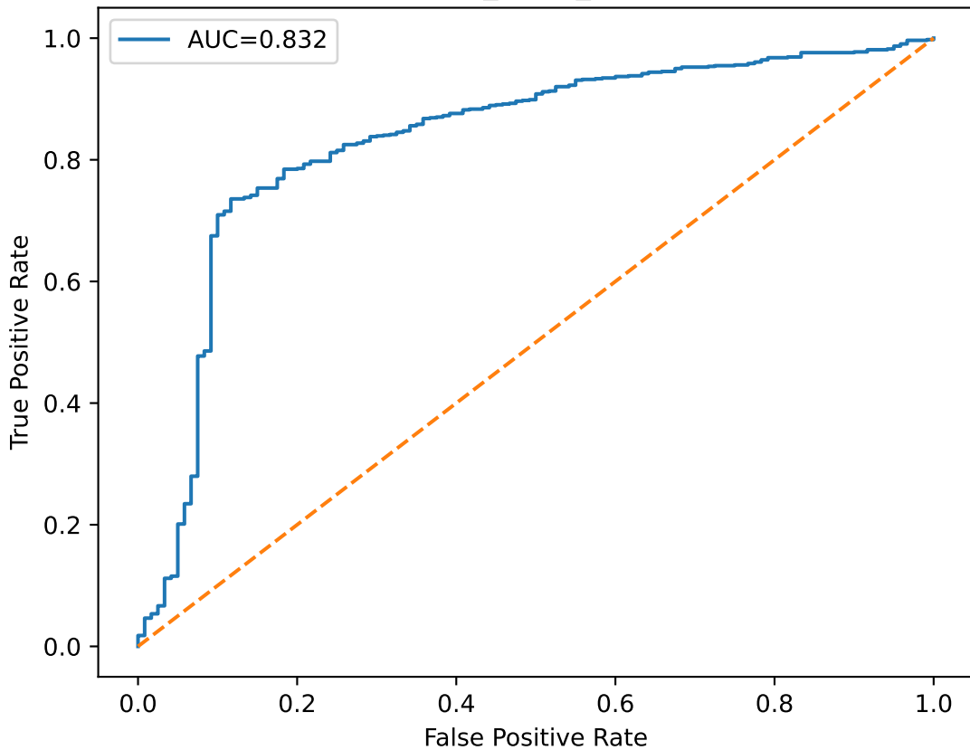
ROC — tfqkd_asym_autoencoder
