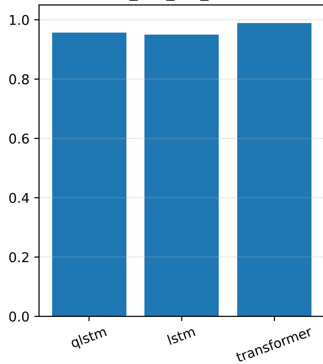
roc_auc_ovr_macro
