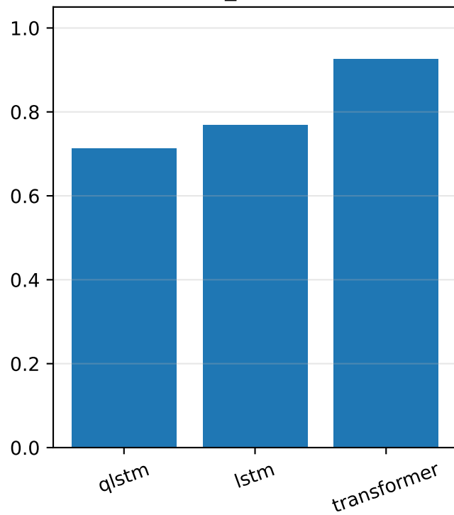
f1_macro
