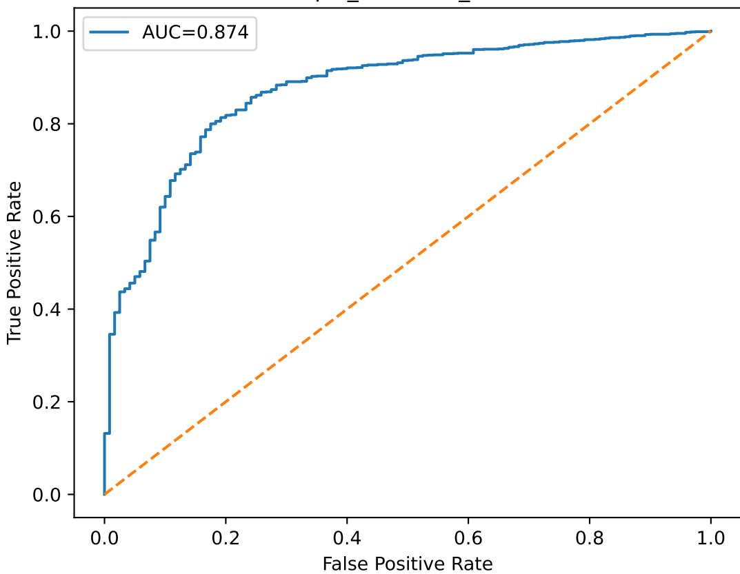
ROC — tfqkd_unknown_autoencoder
