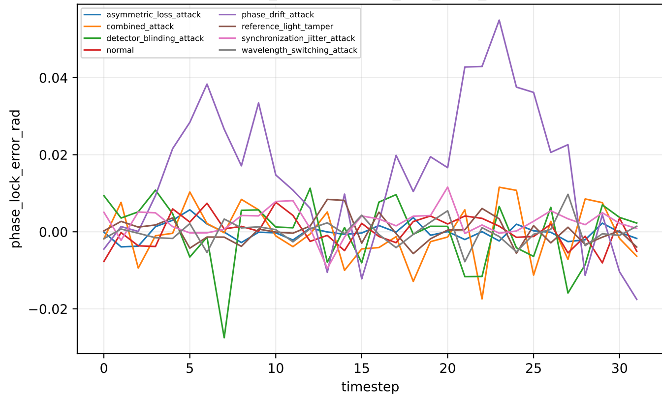
tfqkd_clean — phase_lock_error_rad
