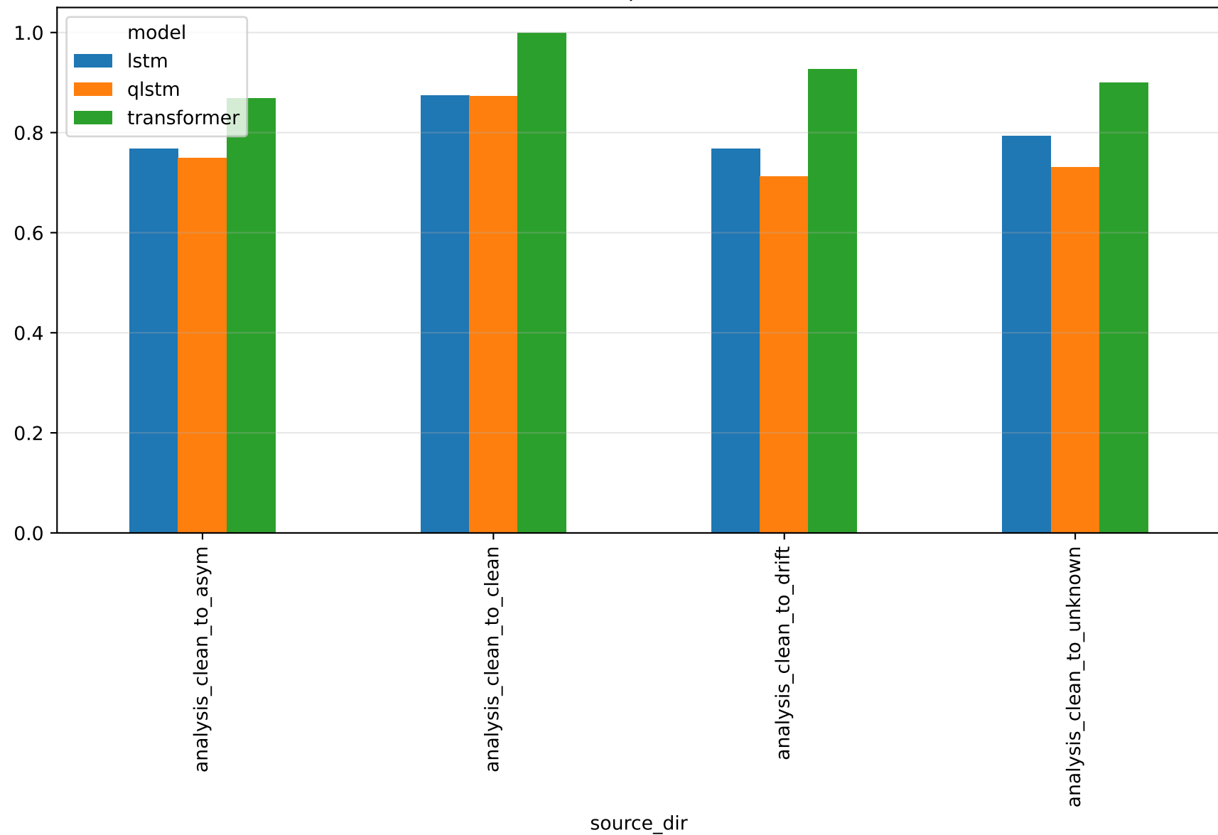
Cross-domain supervised F1 macro
