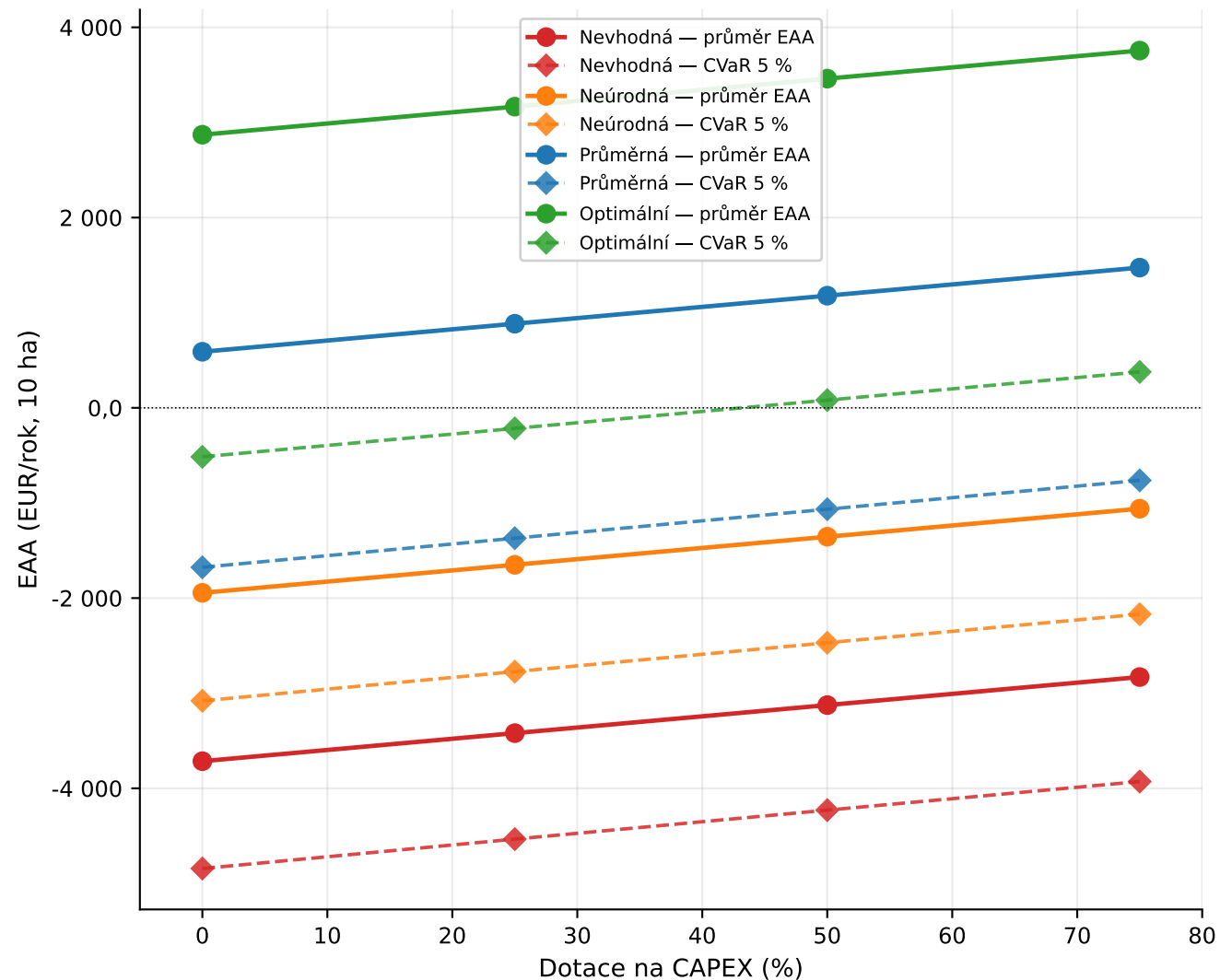
Miscanthus: EAA (—) a CVaR 5 % (- -)
