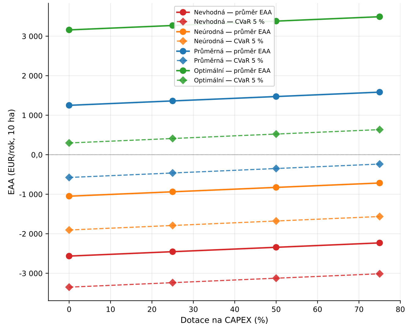
RRD vrba: EAA (—) a CVaR 5 % (- -)
