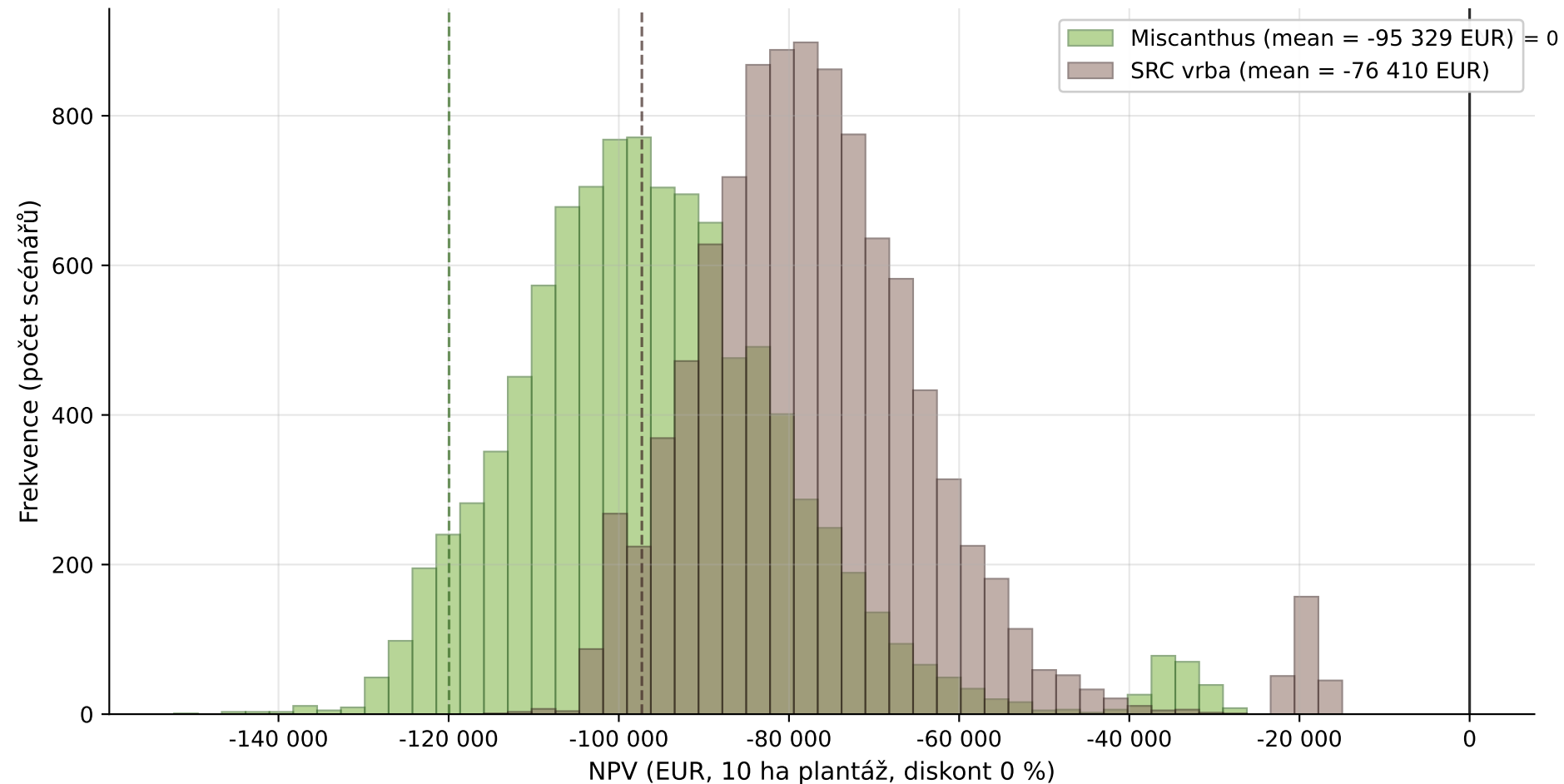
Distribuce NPV — Nevhodná půda (Miscanthus 0-4, SRC 0-4 t DM/ha/rok)
