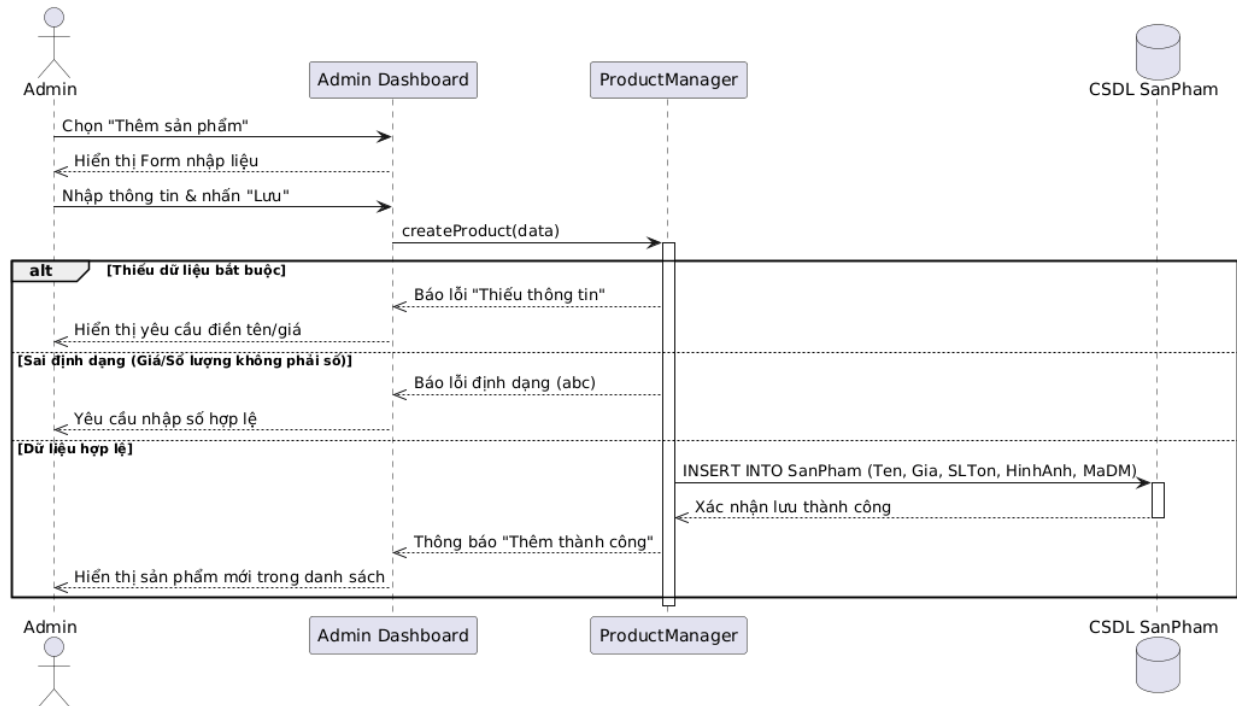
Hình 3. 12: Sequence diagram Thêm sản phẩm mới
