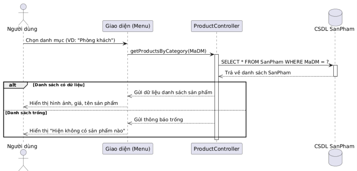
Hình 3. 4: Sequence diagram Xem danh sách sản phẩm
