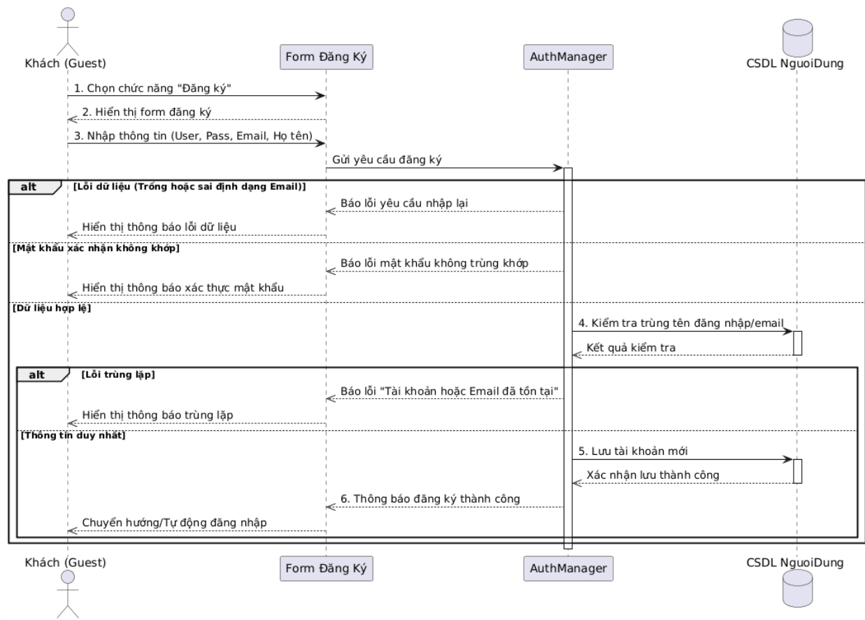
Hình 3. 1: Sequence diagram Đăng ký tài khoản
