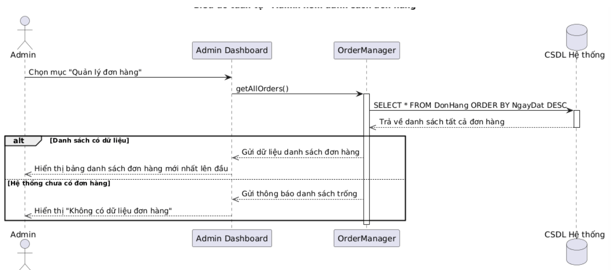
Hình 3. 14: Sequence diagram Xem danh sách đơn hàng
