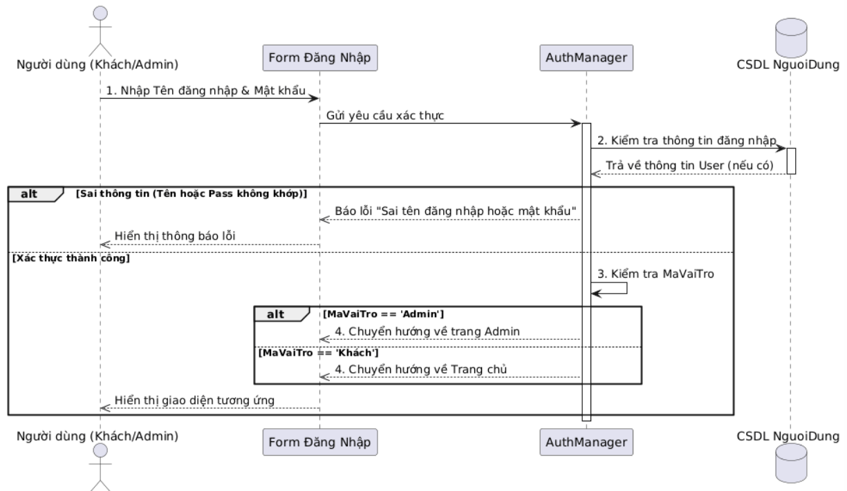
Hình 3. 2: Sequence diagram Đăng nhập
