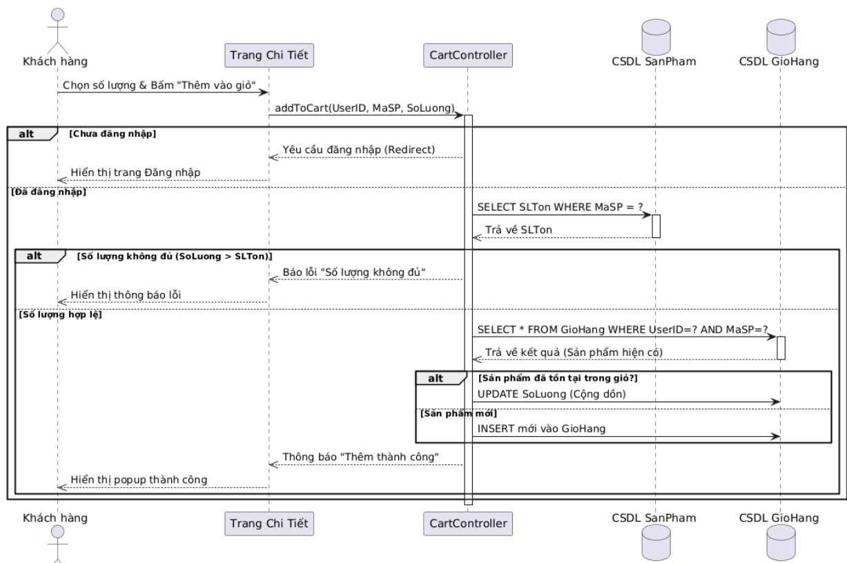
Hình 3. 7: Sequence diagram Thêm vào giỏ
