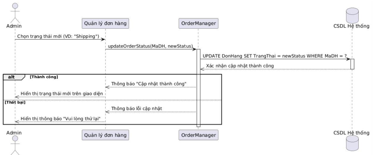
Hình 3. 15: Sequence diagram Cập nhật trạng thái giao hàng
