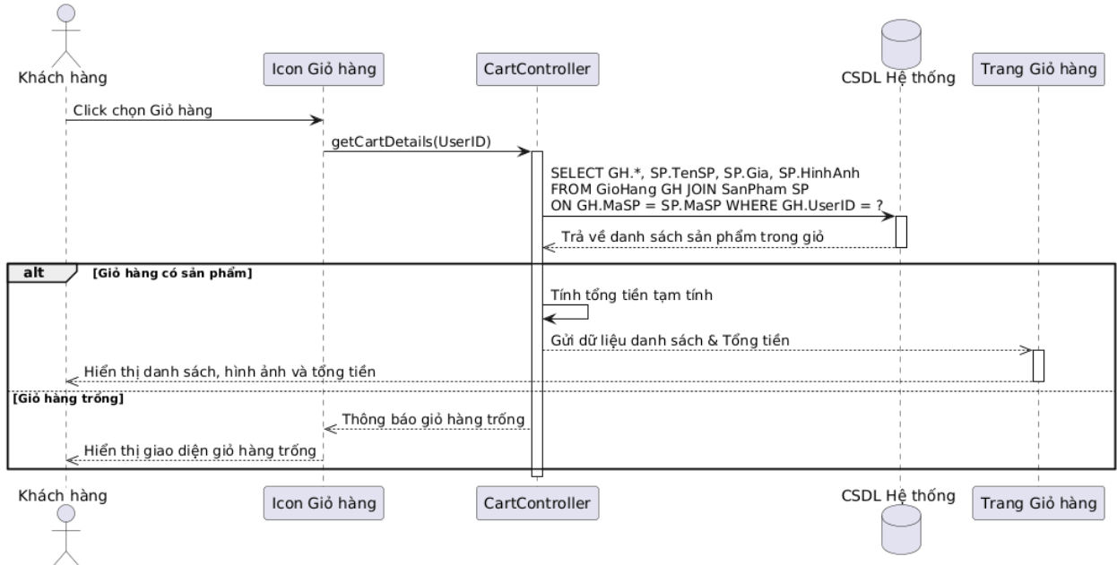
Hình 3. 8: Sequence diagram Xem giỏ hàng
