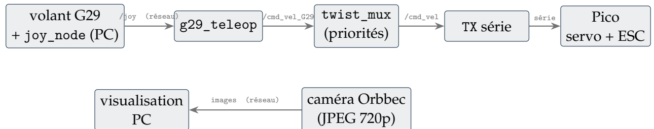
FIGURE 5.1 – Chaîne de téléopération : les commandes descendent du PC vers le véhicule, la vidéo remonte. Les liens marqués « réseau » traversent le WiFi ou la 5G selon la configuration.
