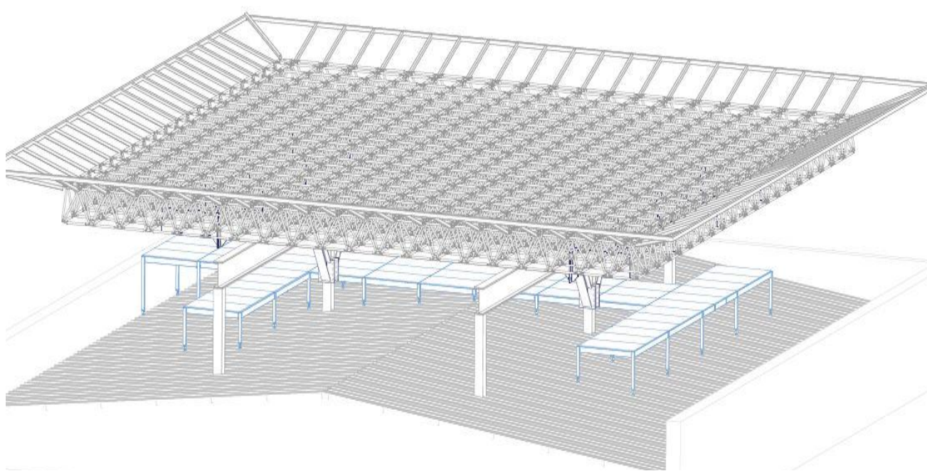
Modelo 3D do projeto estrutural
