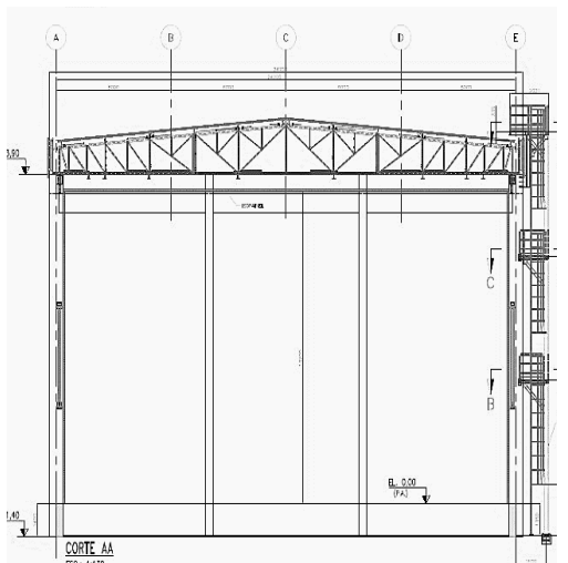
Vista da estrutura
