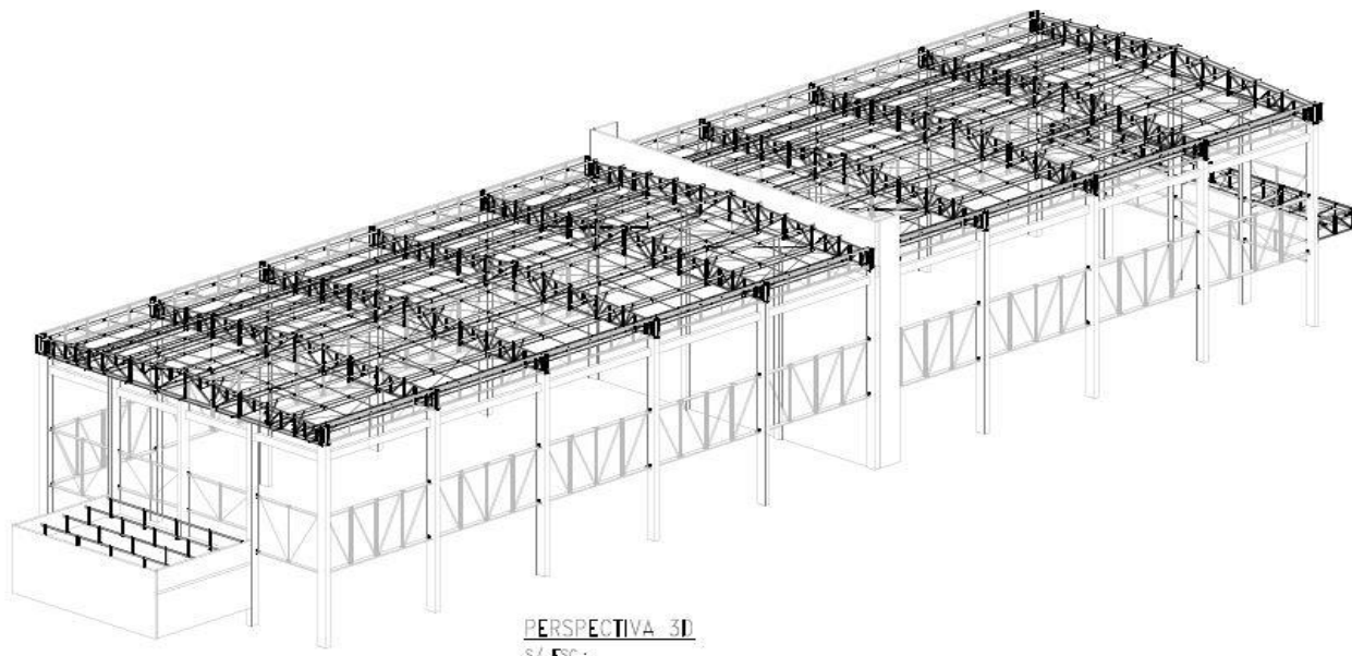
Modelo 3D da estrutura geral do galpão
