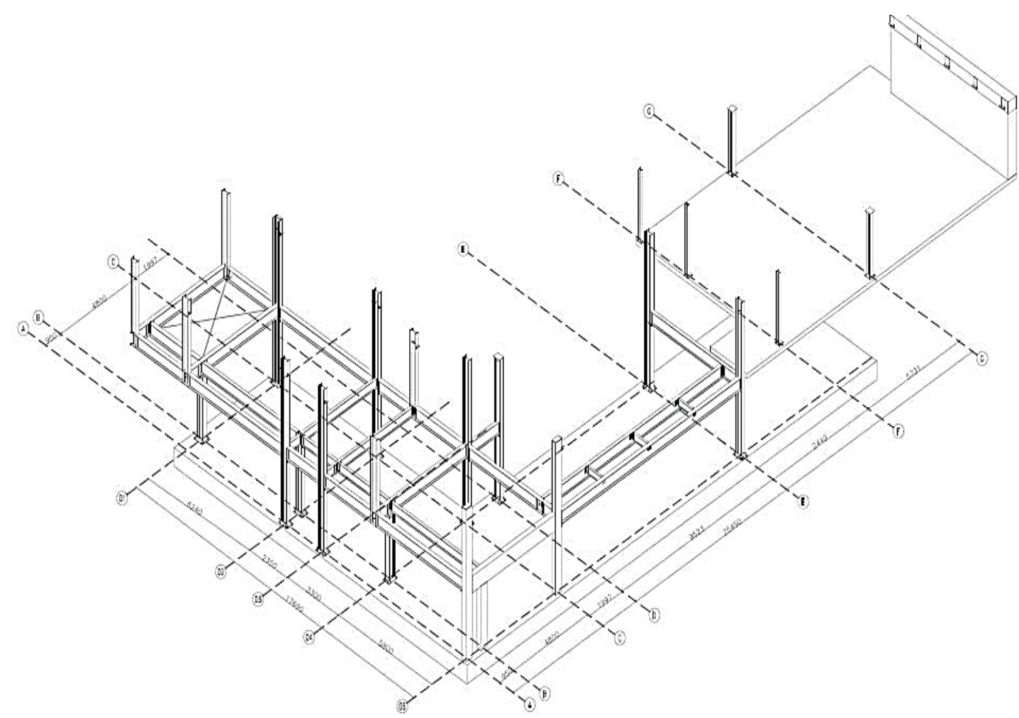
Projeção 3D da estrutura
