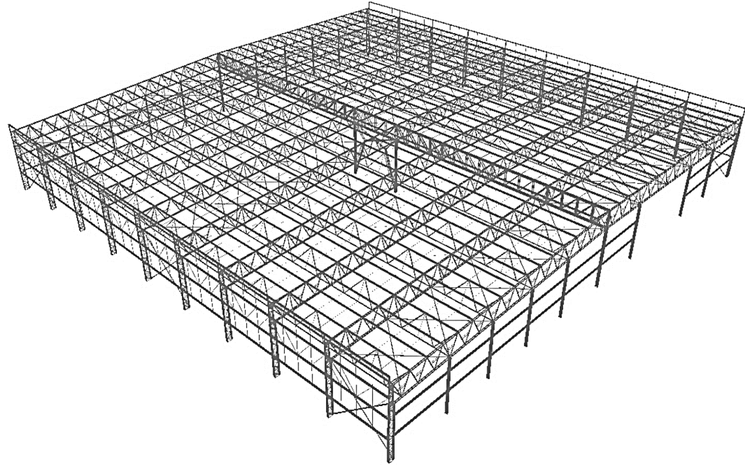
Estrutura metálica do Hangar
