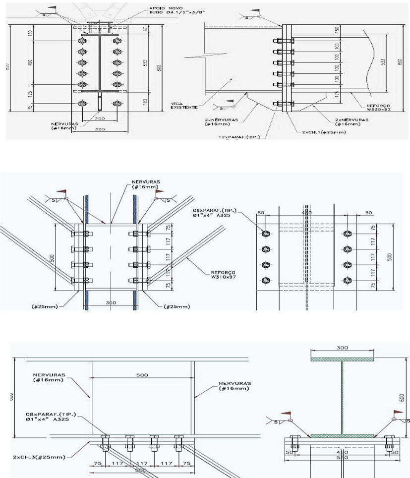
Detalhamentos de encaixes e fixação da estrutura
