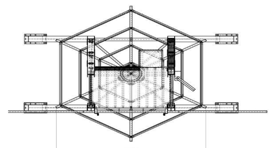
Vista superior da torre
