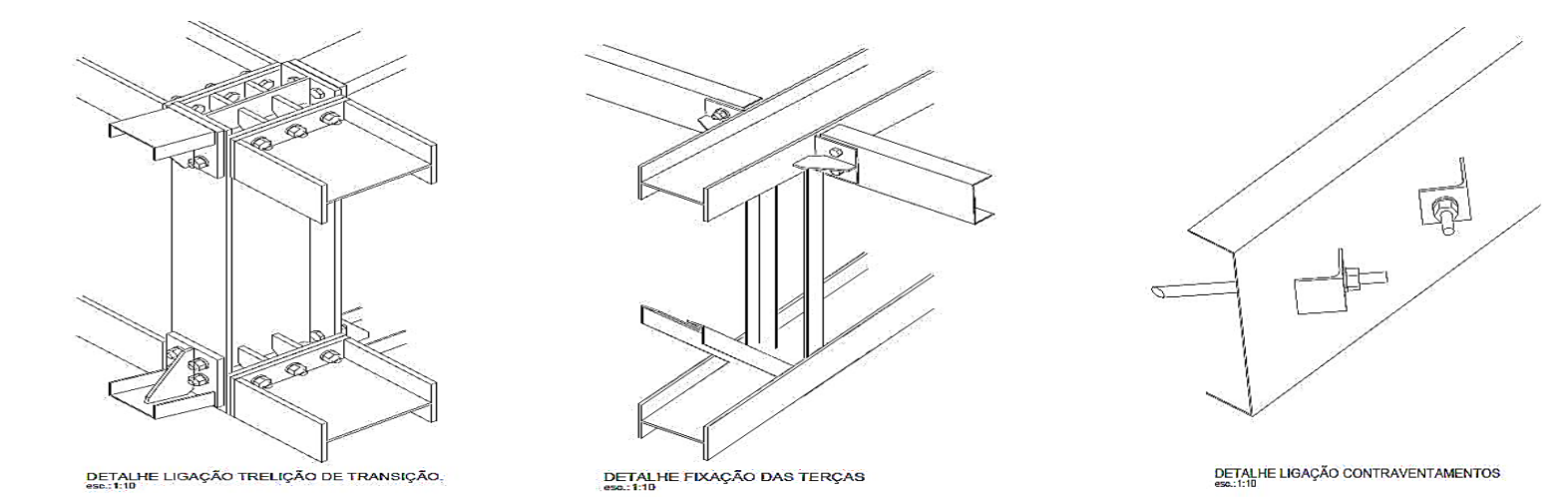
Detalhamento das ligações da estrutura
