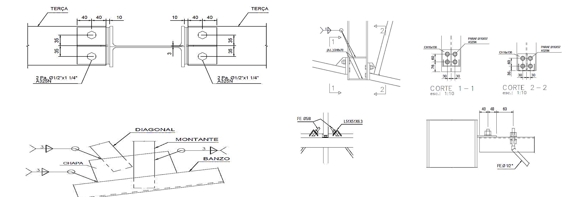
Detalhamentos das ligações da estrutura
