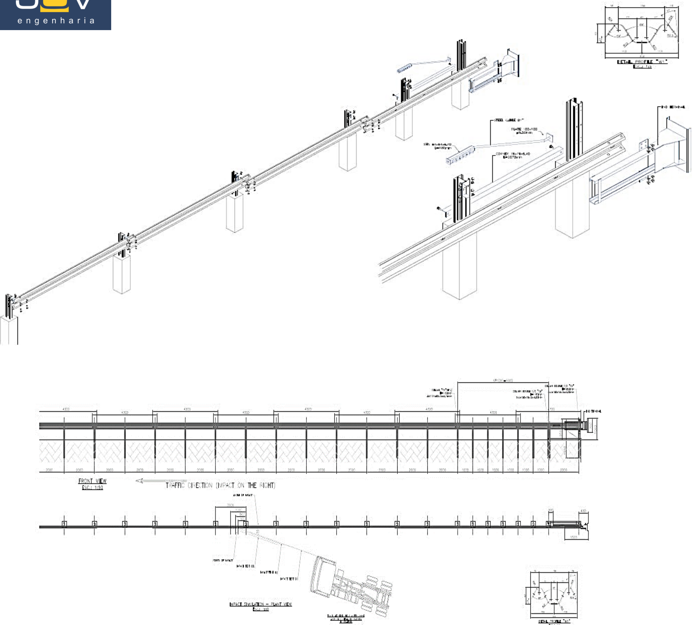
Estrutura geral e simulação de impacto
