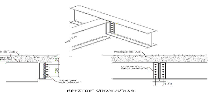
Ligações entre vigas
