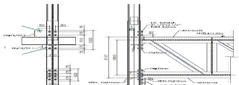
Ligações entre vigas treliçadas
