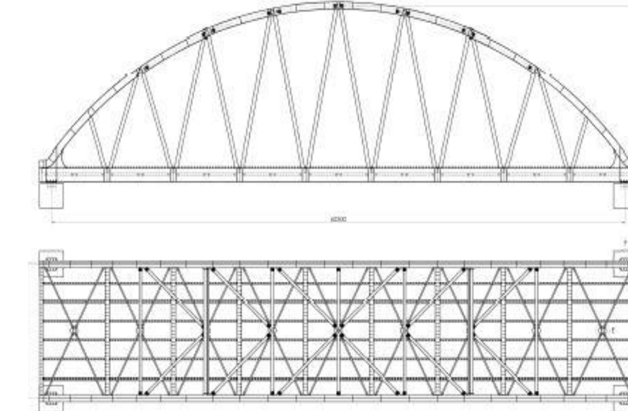
Vista frontal e vista superior da estrutura
