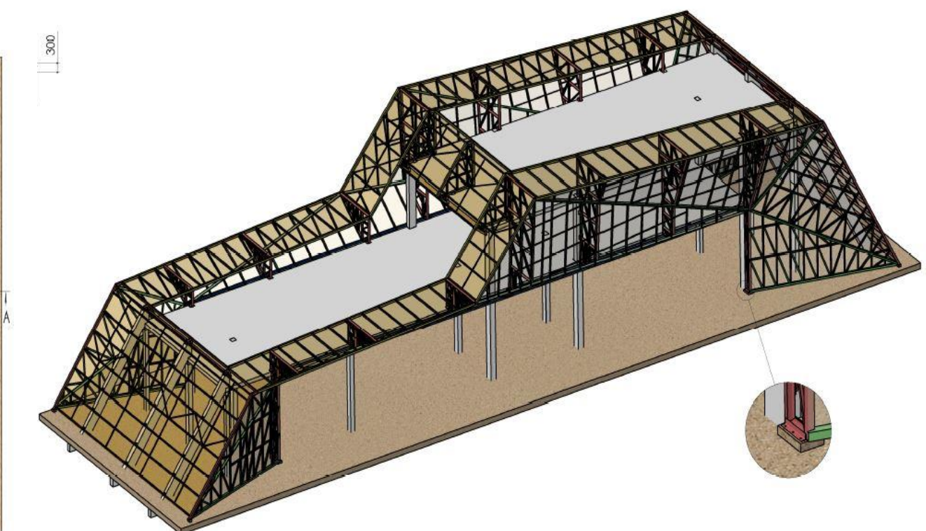
Modelo 3D da estrutura geral da portaria
