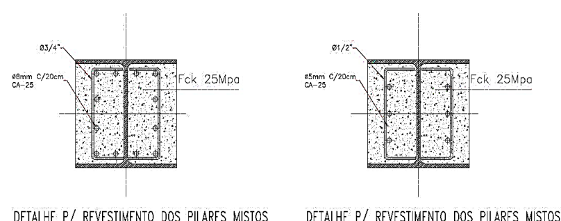
Revestimentos dos pilares mistos
