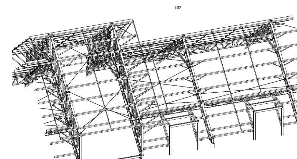
Perspectiva da estrutura da cobertura
