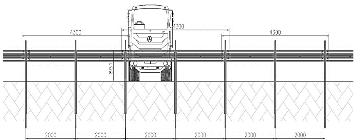
Vista vista frontal da estrutura
