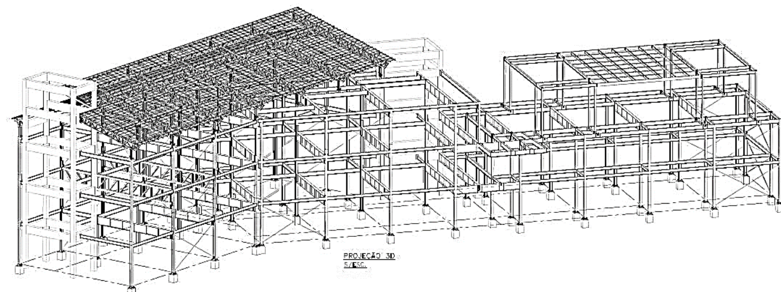
Projeção 3D da estrutura
