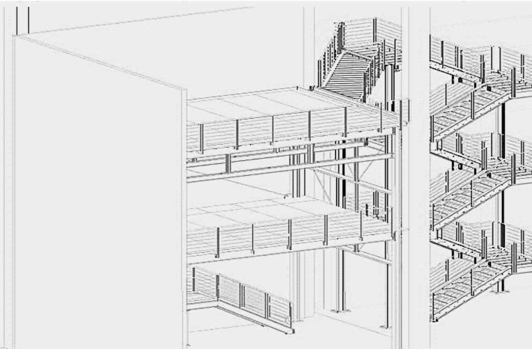
Modelo 3D da estrutura
