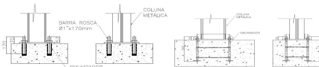
Detalhamento dos chumbadores
