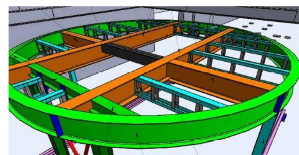
Estrutura metálica em arco para sala reuniões
