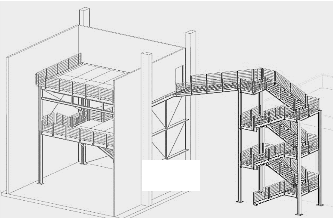
Perspectiva da estrutura
