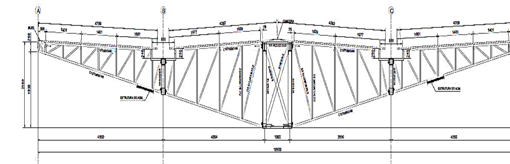
Vista da estrutura da cobertura
