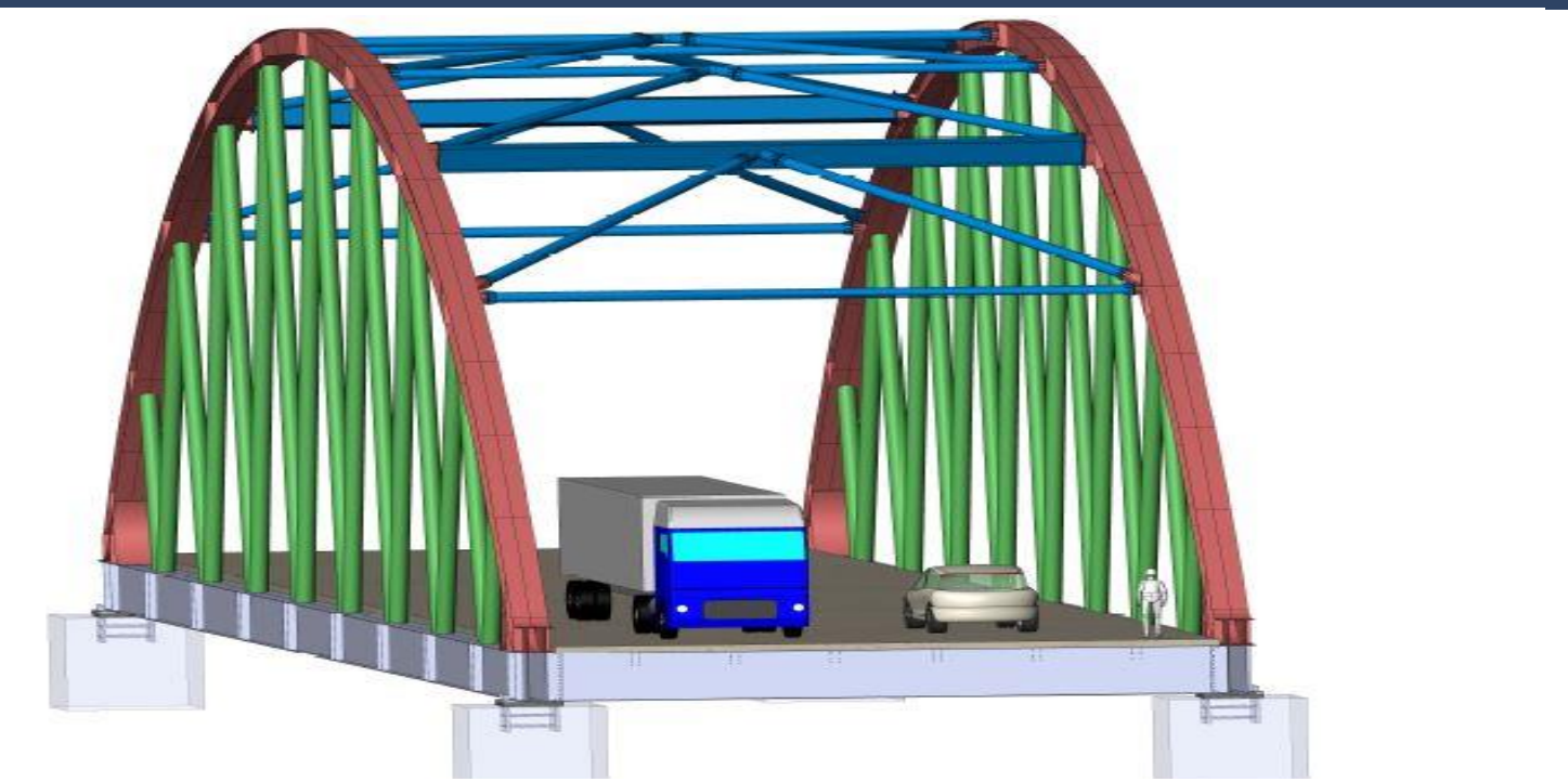
Modelo 3D da estrutura geral da ponte
