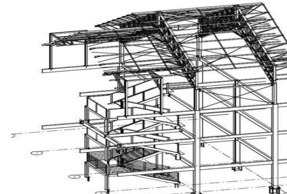
Perspectiva da estrutura do prédio e da escada
