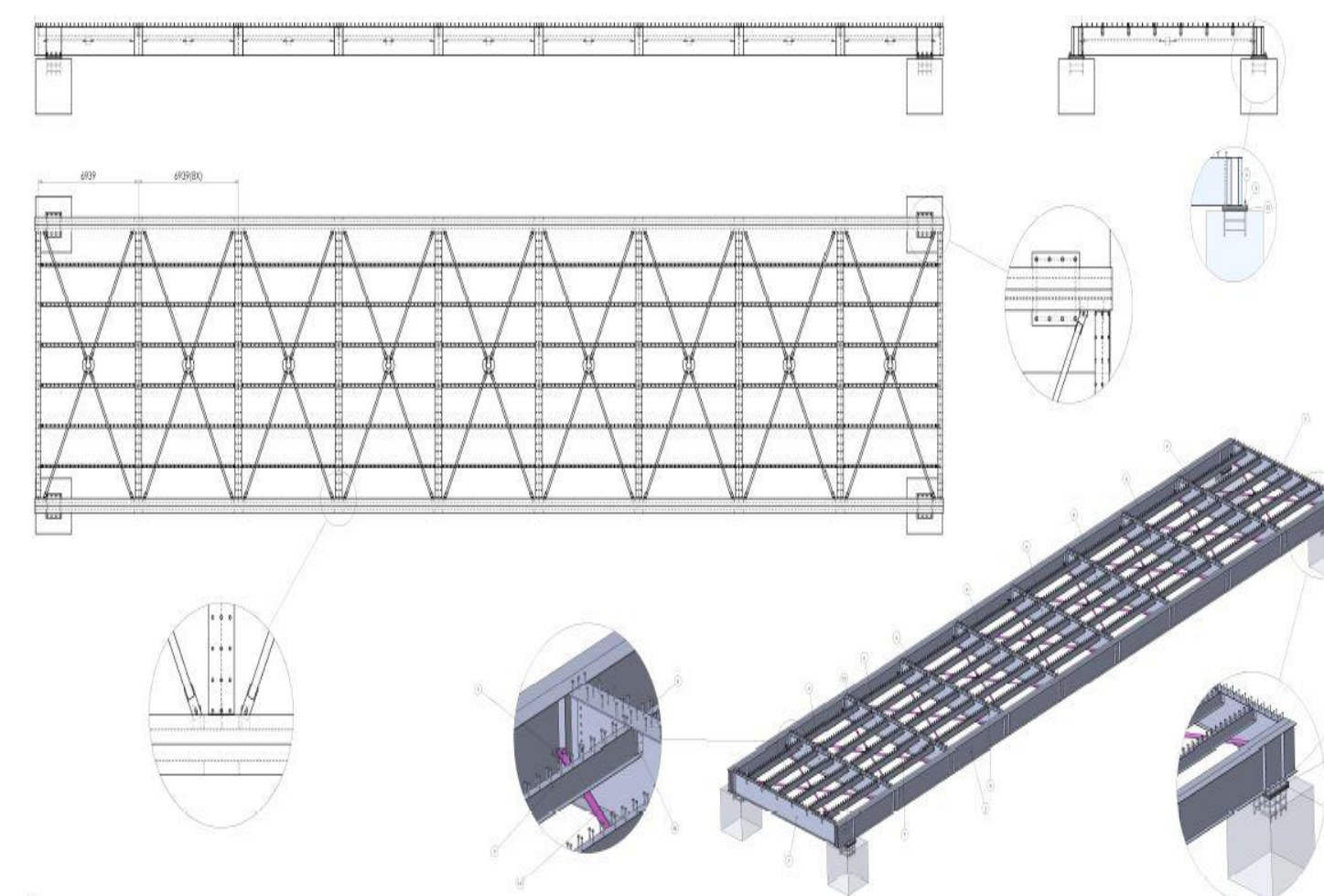
Fixação das travessas, contraventamentos e sapatas
