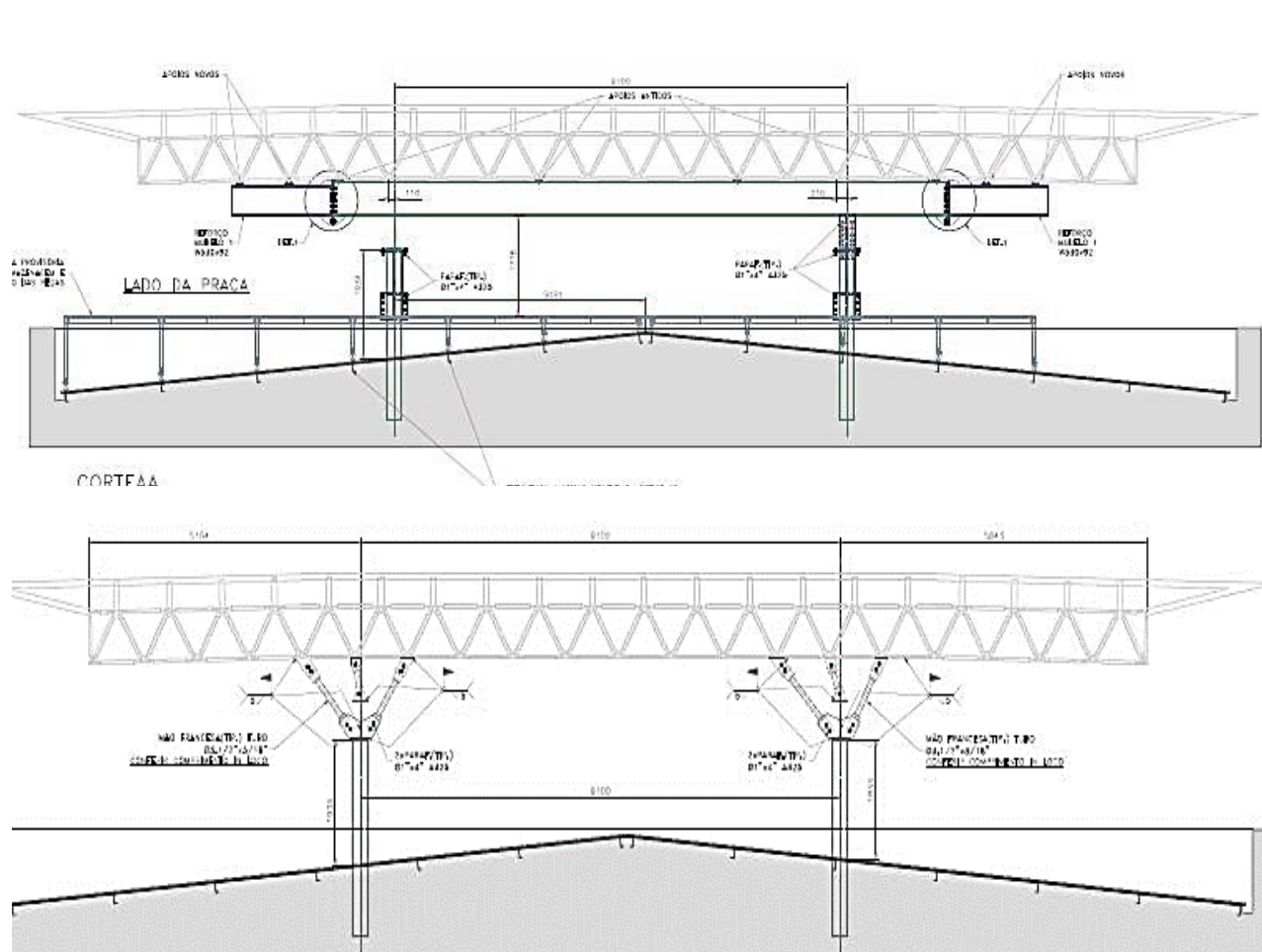
Vistas da estrutura metálica
