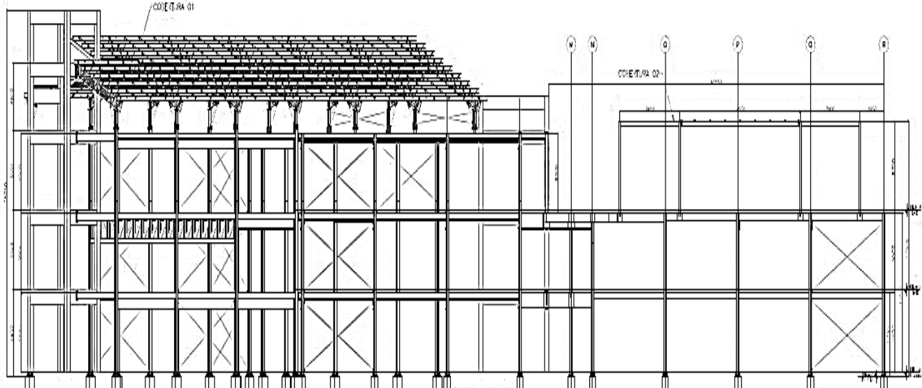
Vista frontal da estrutura
