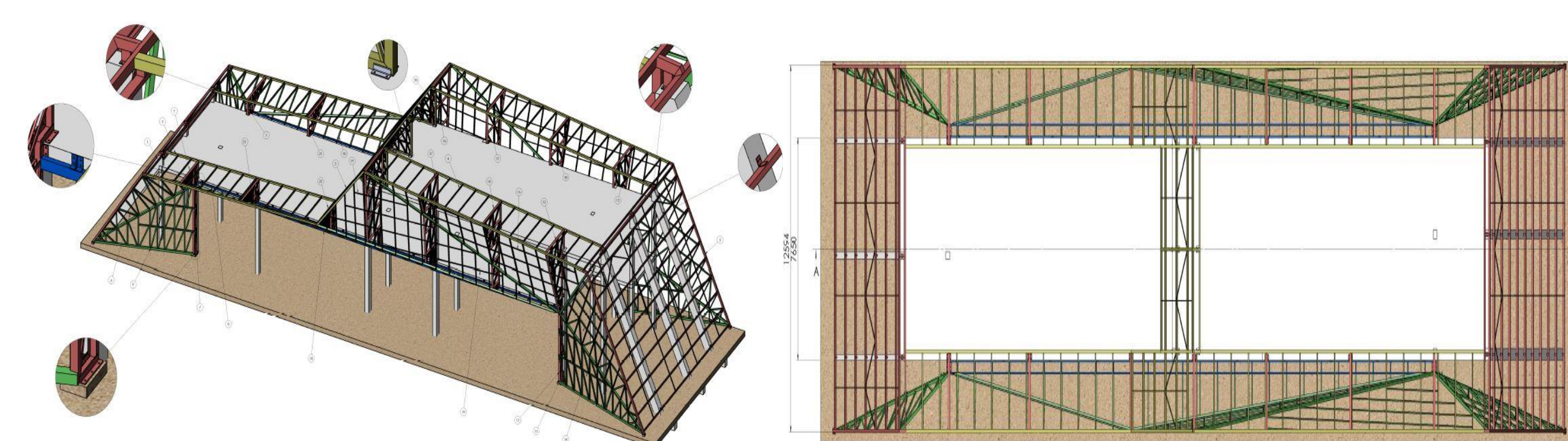
Indicações das fixações da estrutura
