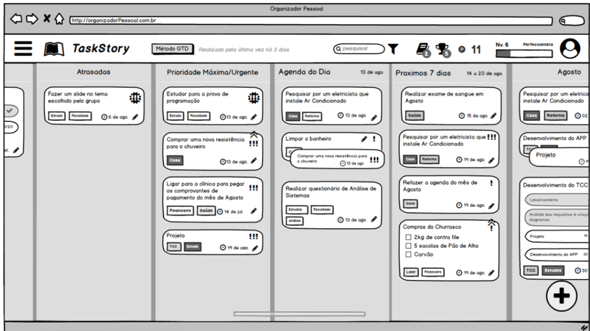
Figura 9 – Protótipo de interface do painel principal da aplicação.
