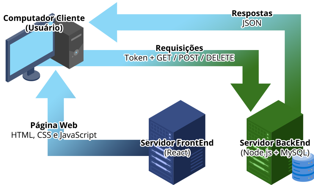
Figura 20 – Esquema simples da comunicação da arquitetura Cliente-Servidor.
