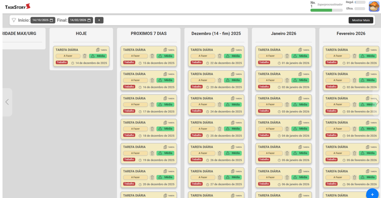
Figura 25 – Validação do algoritmo de recorrência no frontend : o componente Panel renderiza múltiplas instâncias visuais (cards) a partir de um único registro JSON, demonstrando a eficiência na gestão de memória do navegador.
