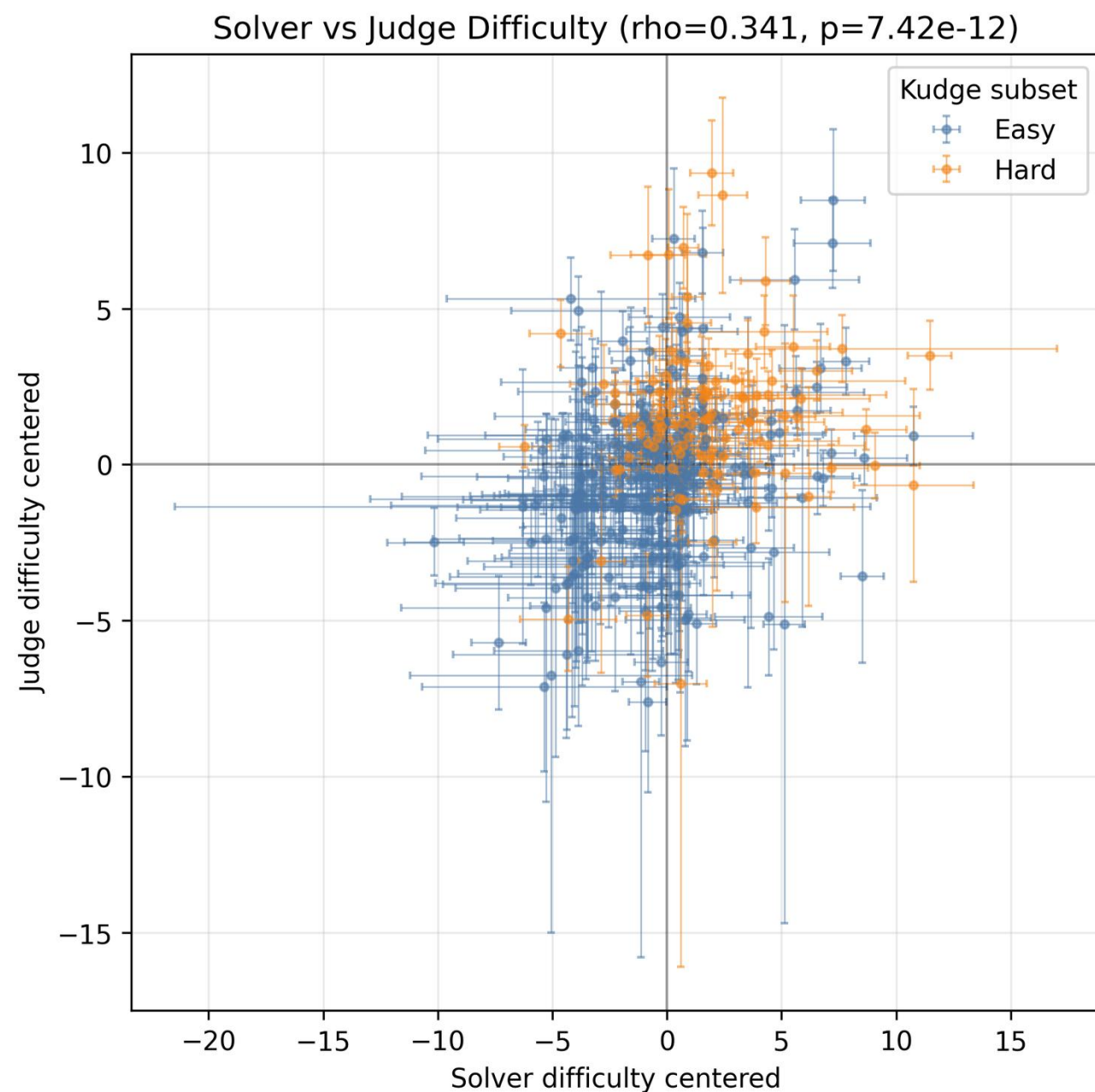
A. Korean QA (KUDGE, K=2)
