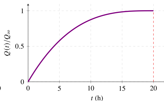
Figura A.13: Exercício ??: O gráfico apresenta o perfil cinético cúbico de erosão até o esgotamento em t = 20 h.
