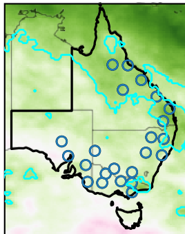
d) Dec ENSO
