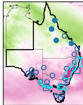
f) Sep SAM
