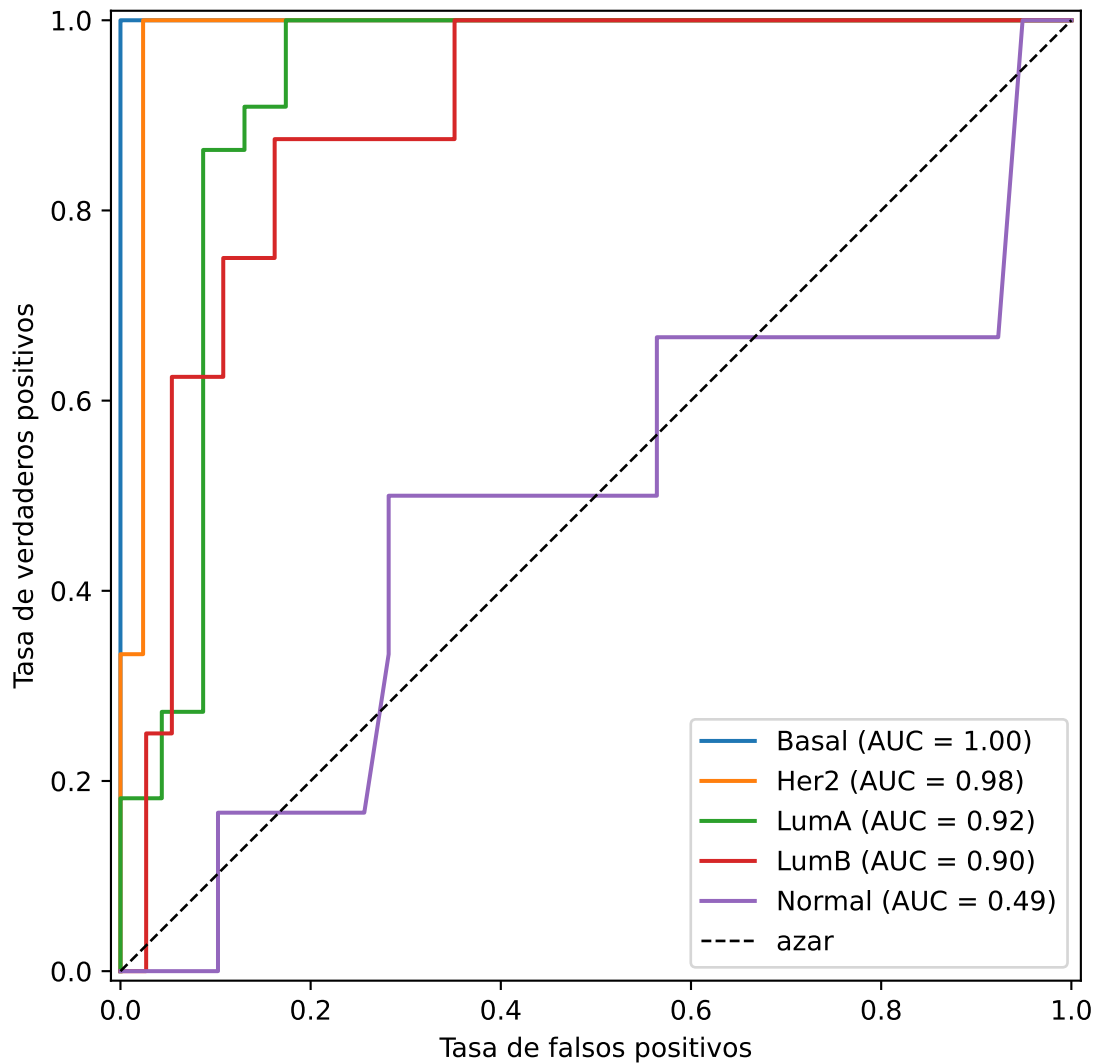
Curvas ROC (cada clase contra el resto) AUC macro=0.857
