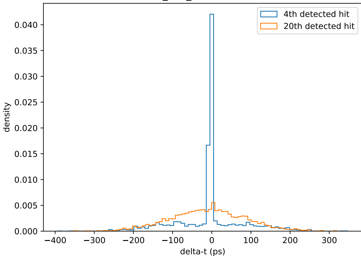
POS_REF_2: x=-443 mm
