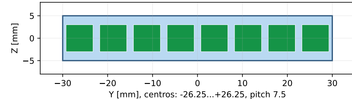
Config End: una cara \pm X (vista Y-Z), IDs 0-7 / 8-15
