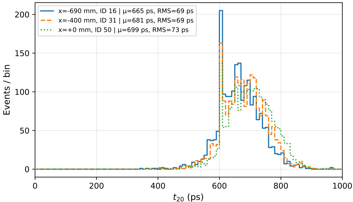
F1 — EJ-230 t_{20} top-nearest, absolute counts (2000 evt/run)
