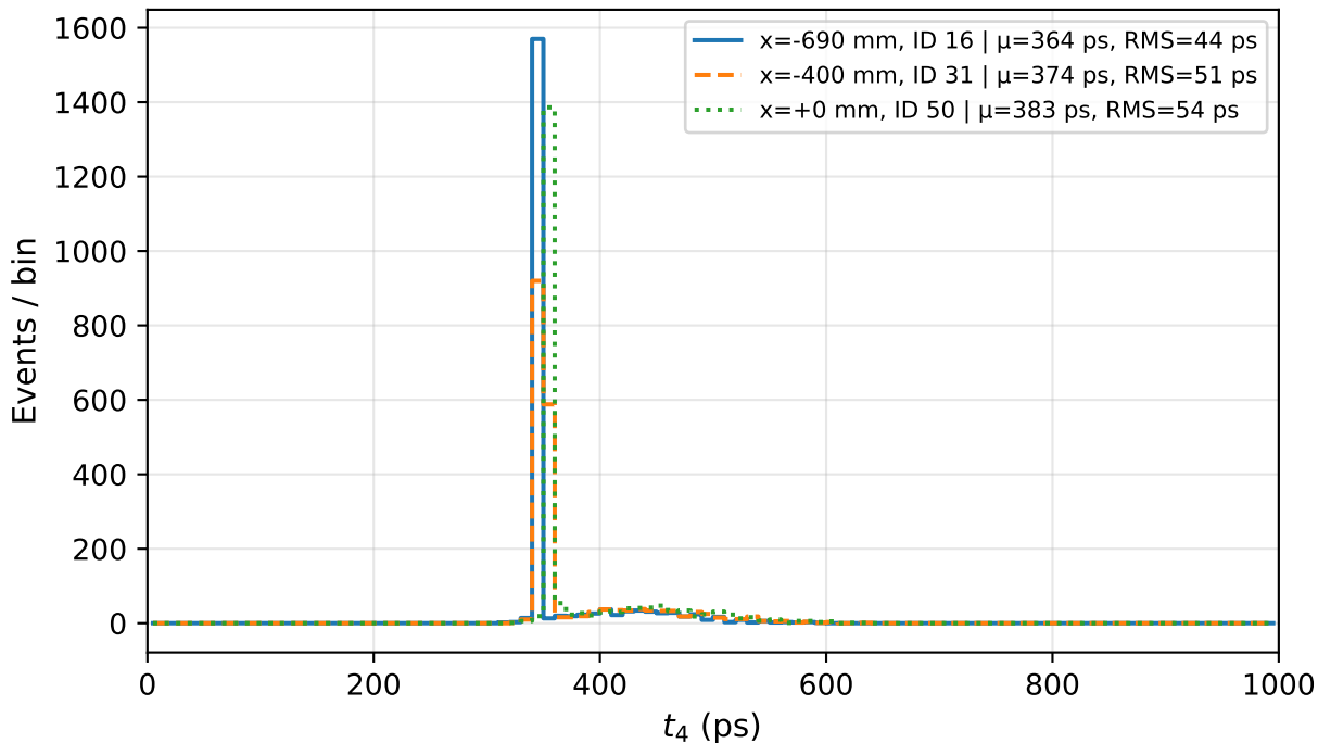
F1 — EJ-230 t_4 top-nearest, absolute counts (2000 evt/run)
