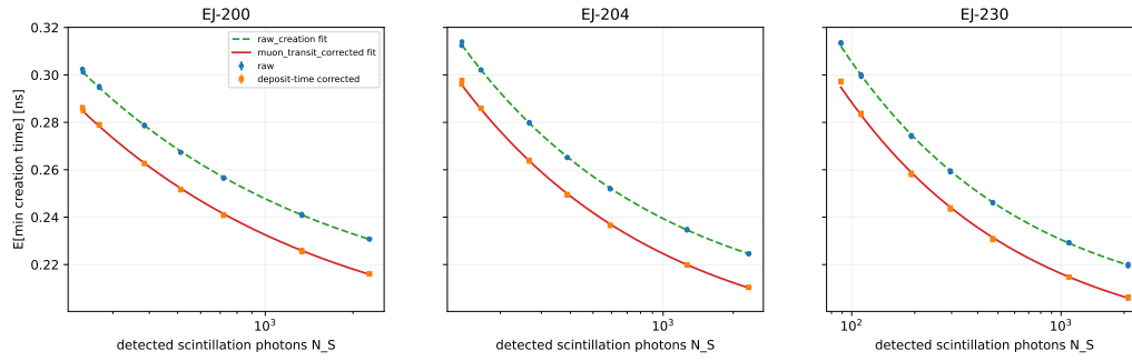
Figure 6.3: Corrección por tránsito del muón.
