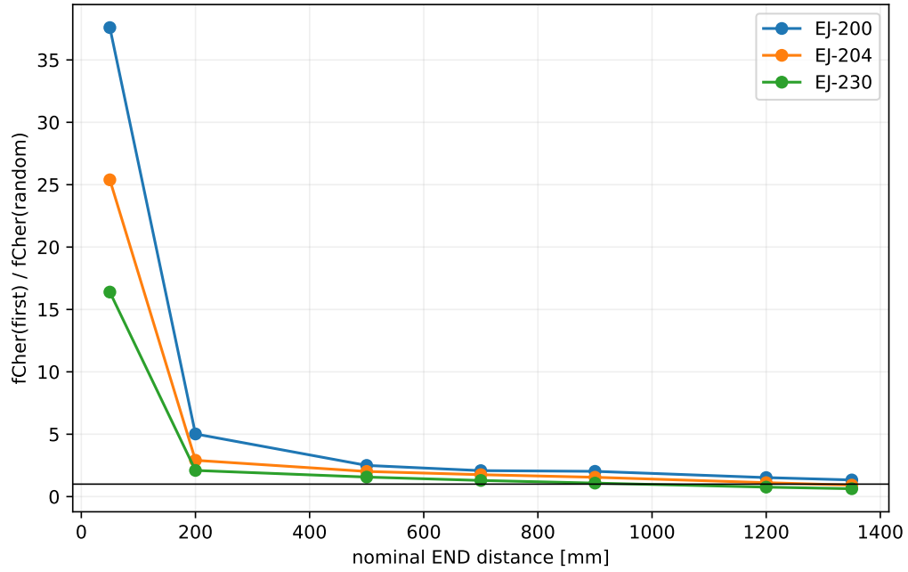
Figure 8.4: Enriquecimiento en v2.
