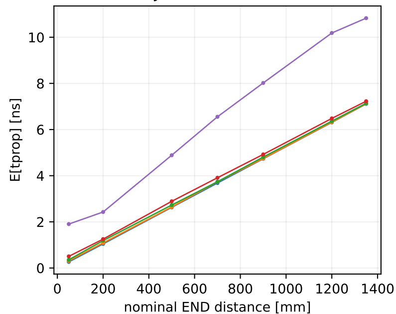
EJ-200, Cherenkov
