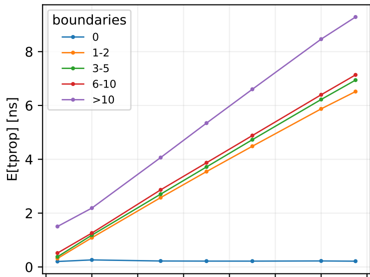
EJ-200, scintillation
