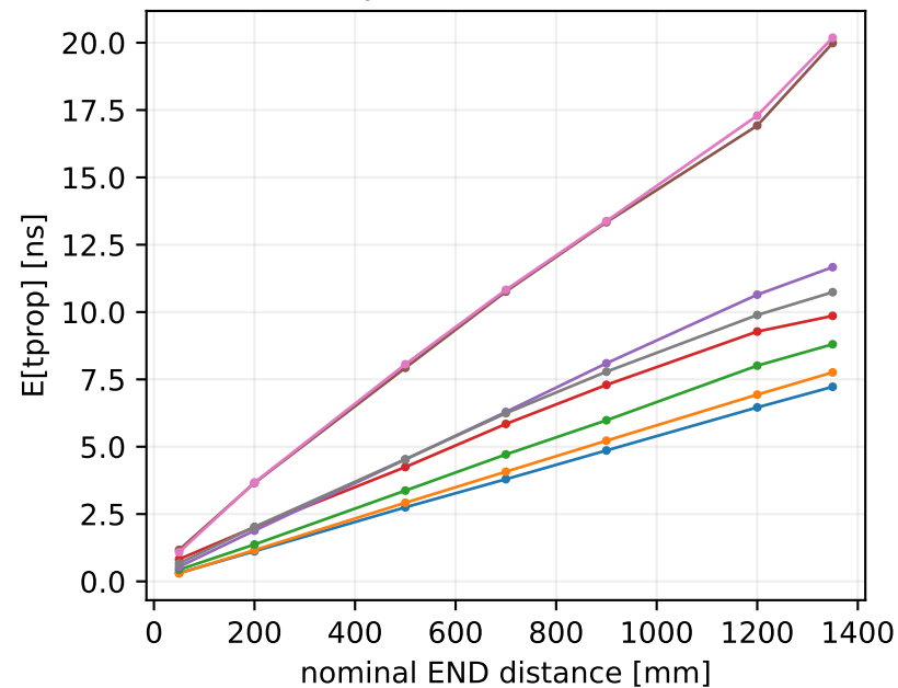
EJ-200, Cherenkov
