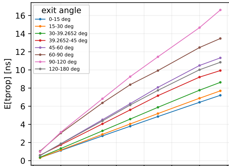
EJ-200, scintillation
