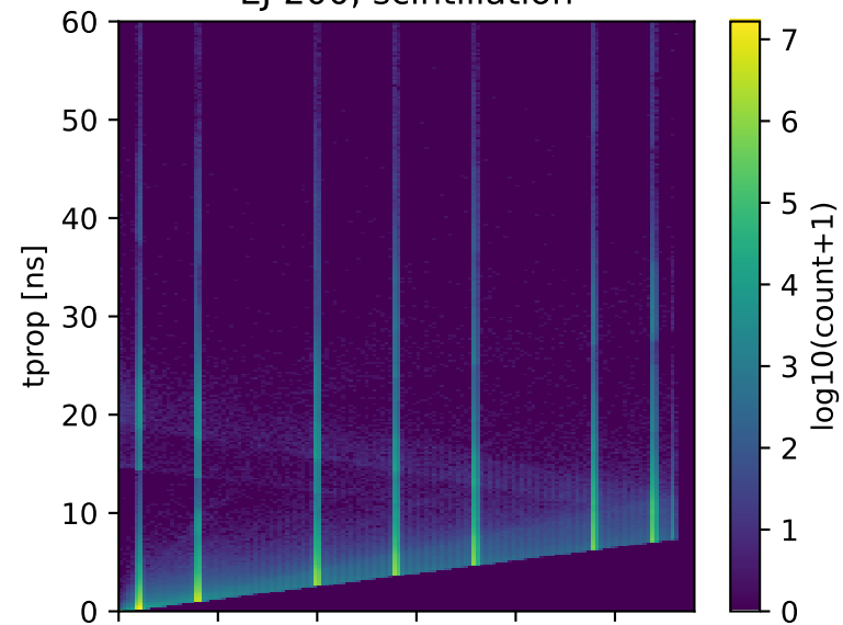
EJ-200, scintillation
