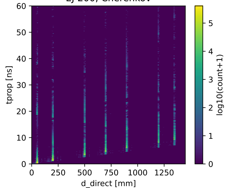
EJ-200, Cherenkov
