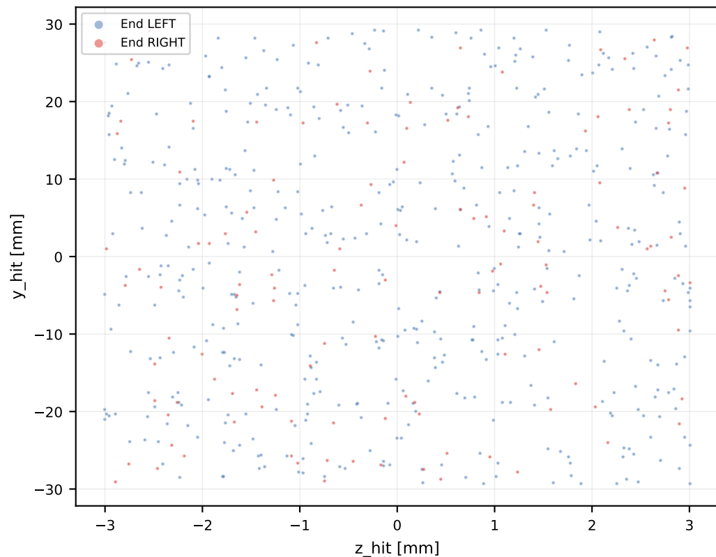
Transverse section (z vs y) EJ-204 x gun =+0 mm
