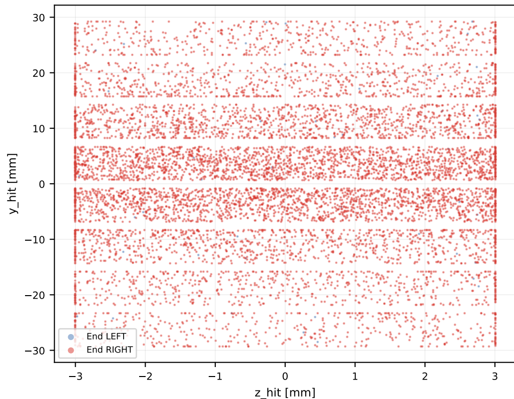
Transverse section (z vs y) EJ-204 x gun =+690 mm
