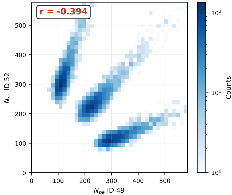
Pair A: IDs 49/52 (X=-32mm / +32mm, sep 64mm) (sep=64 mm)
