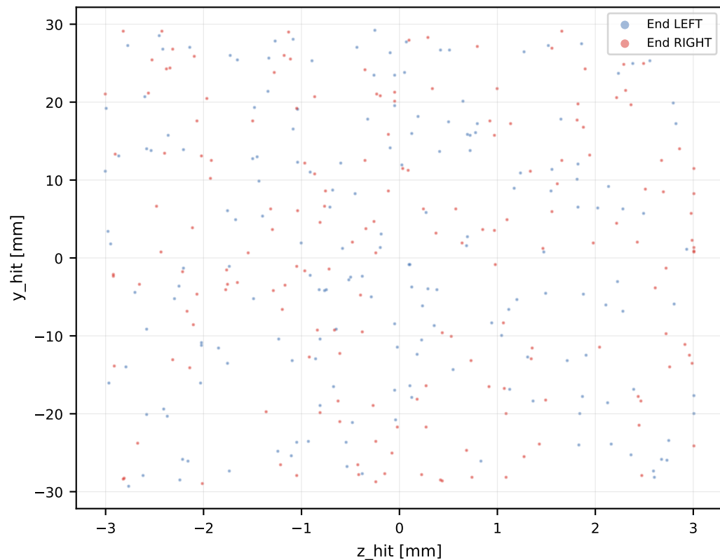
Transverse section (z vs y) EJ-230 x gun =+0 mm
