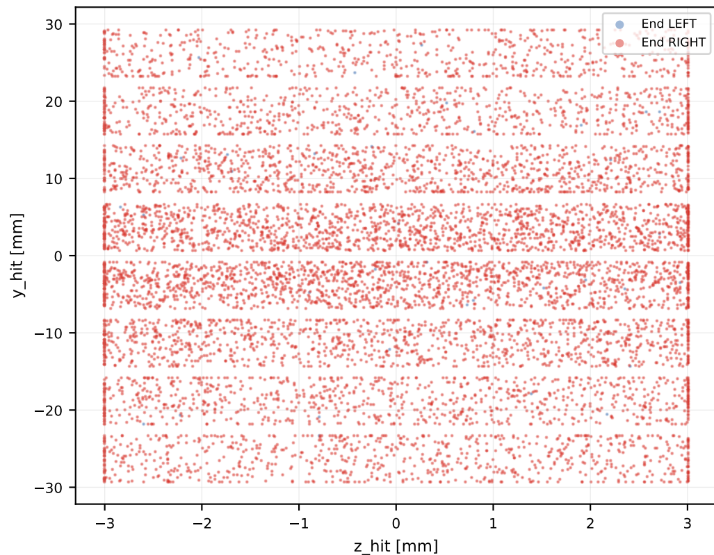
Transverse section (z vs y) EJ-230 x_gun=+690 mm
