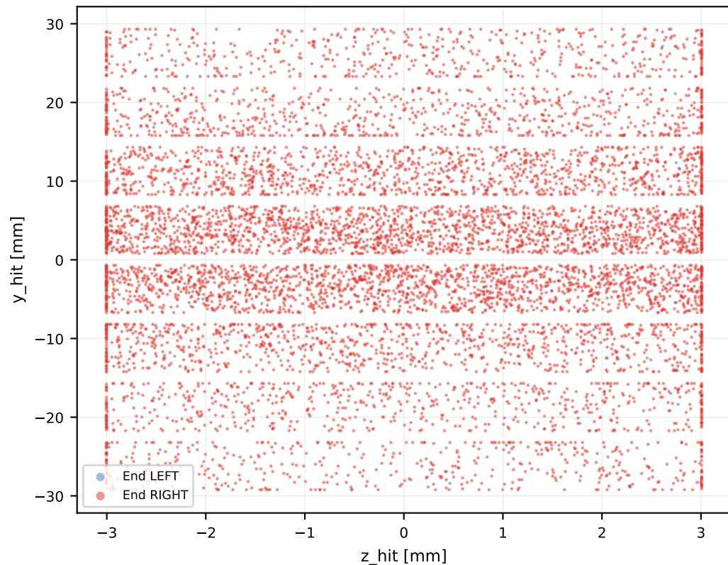
Sección transversal (z vs y) EJ-204 x_gun=+690 mm
