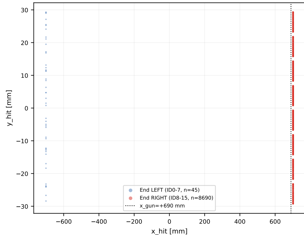
Vista longitudinal (x vs y) EJ-204 x_gun=+690 mm ev=1415
