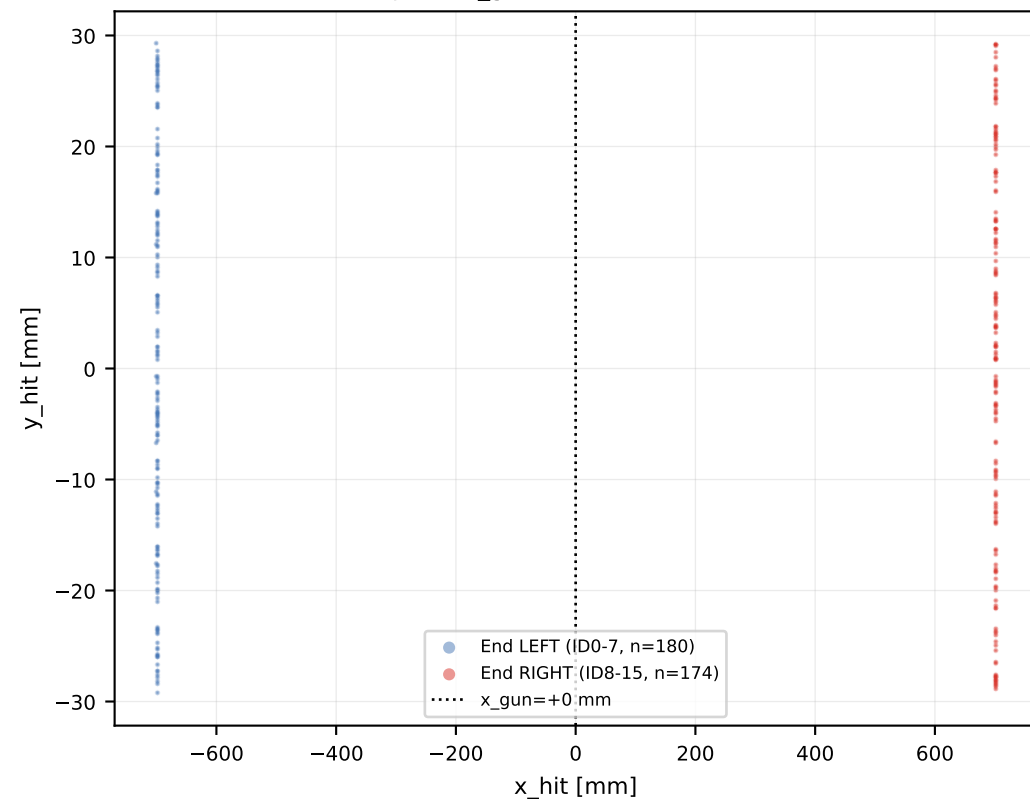
Vista longitudinal (x vs y) EJ-230 x_gun=+0 mm ev=1546
