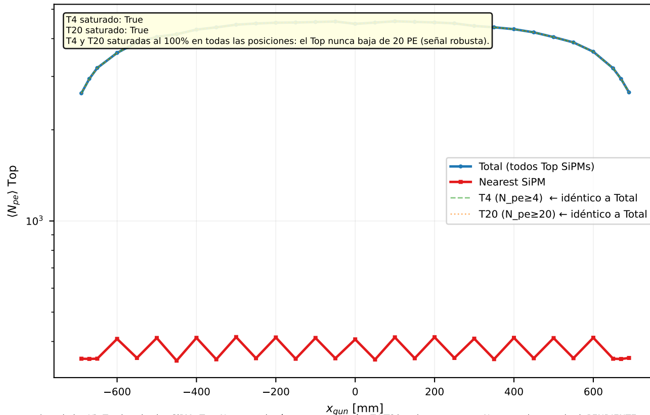
F4 — Perfiles N_{pe} Top vs posición (EndTop EJ-204, log-Y)
