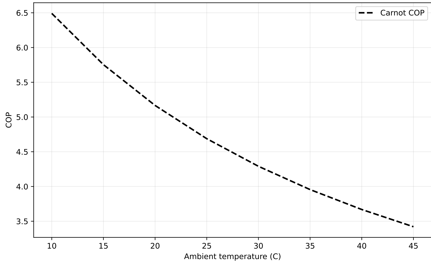
R134a: IDAES NTU PLR + HX vs Carnot
