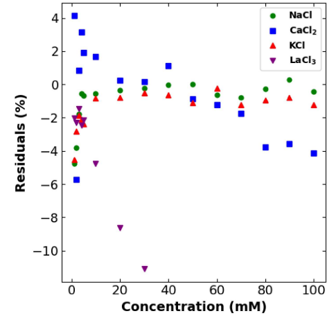
(d) Percent error of the MSA model
