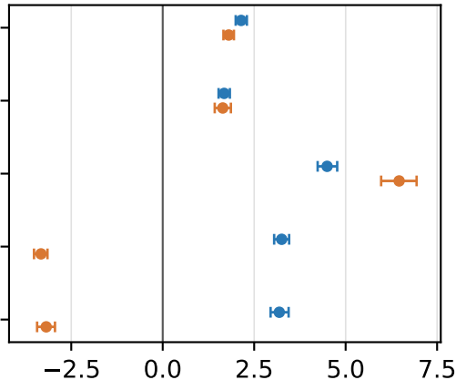
Qwen3-8B
