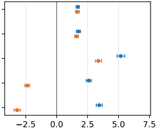
Gemma 3 4B
