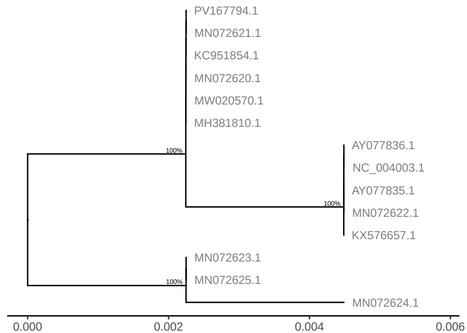
GTPV gene LSDV117
