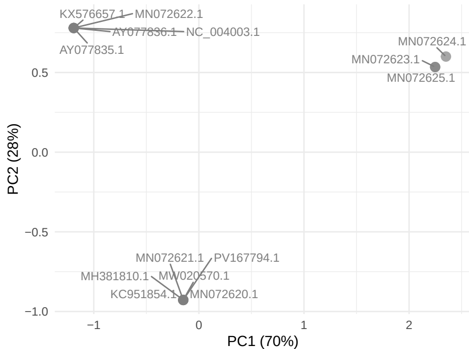
GTPV gene LSDV117
