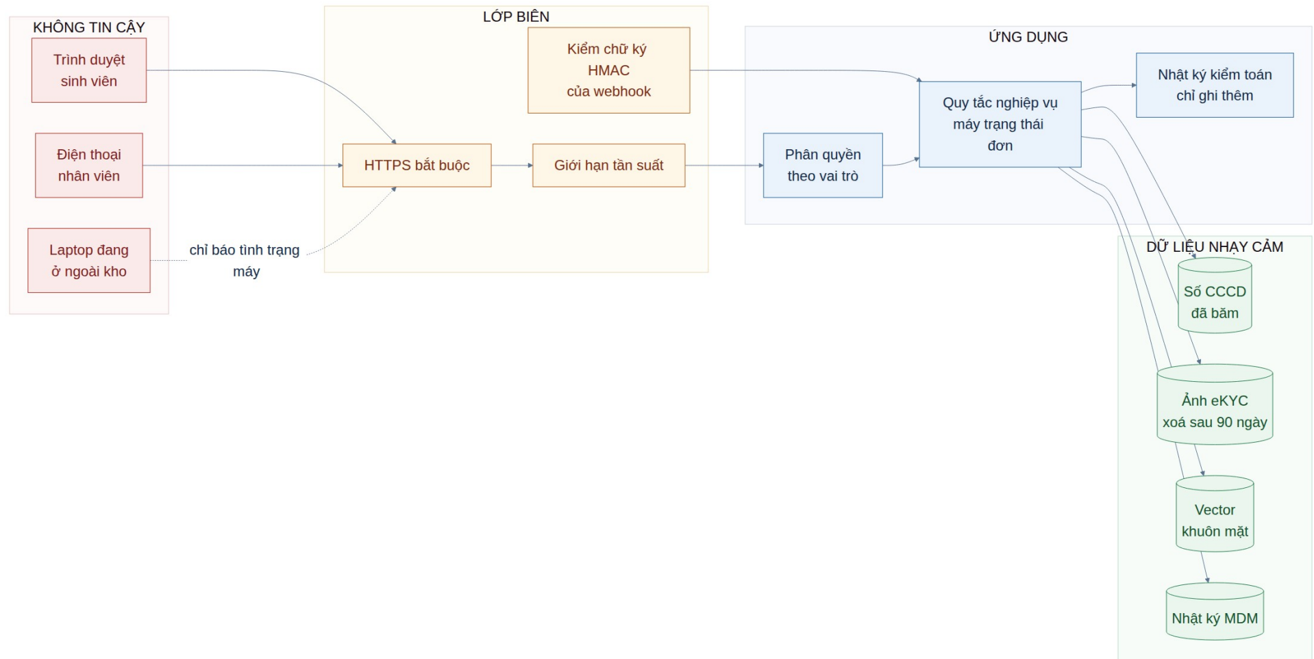
Hình 10. Bốn vùng tin cậy của hệ thống ExamLap và những thứ được phép đi qua từng ranh giới.
