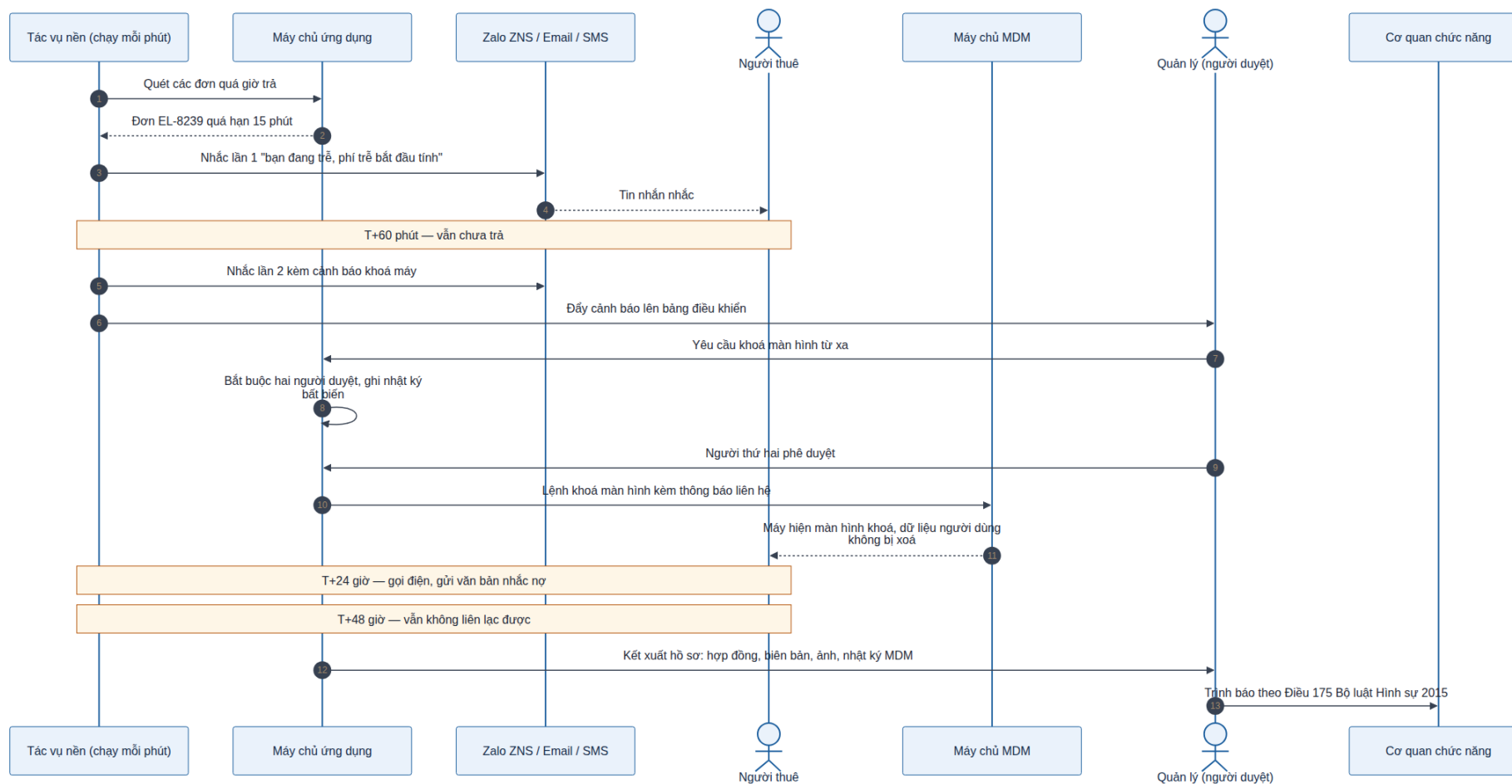
Hình 9. Trình tự xử lý đơn thuê quá hạn: năm mốc thời gian từ nhắc tự động tới trình báo, với điểm chốt hai người duyệt trước khi phát lệnh khoá màn hình.
