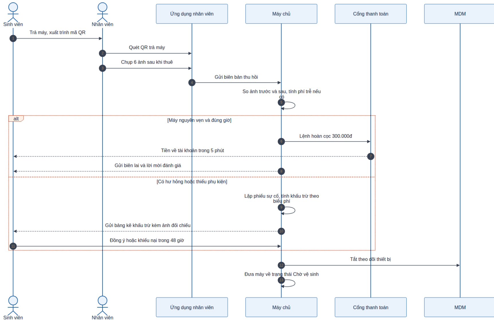
Hình 18. Trình tự trả máy và hoàn cọc với hai nhánh: máy nguyên vẹn thì lệnh hoàn cọc ba trăm nghìn đồng chạy trong năm phút, còn có hư hỏng thì lập phiếu sự cố và gửi bảng kê khấu trừ kèm ảnh đối chiếu.
