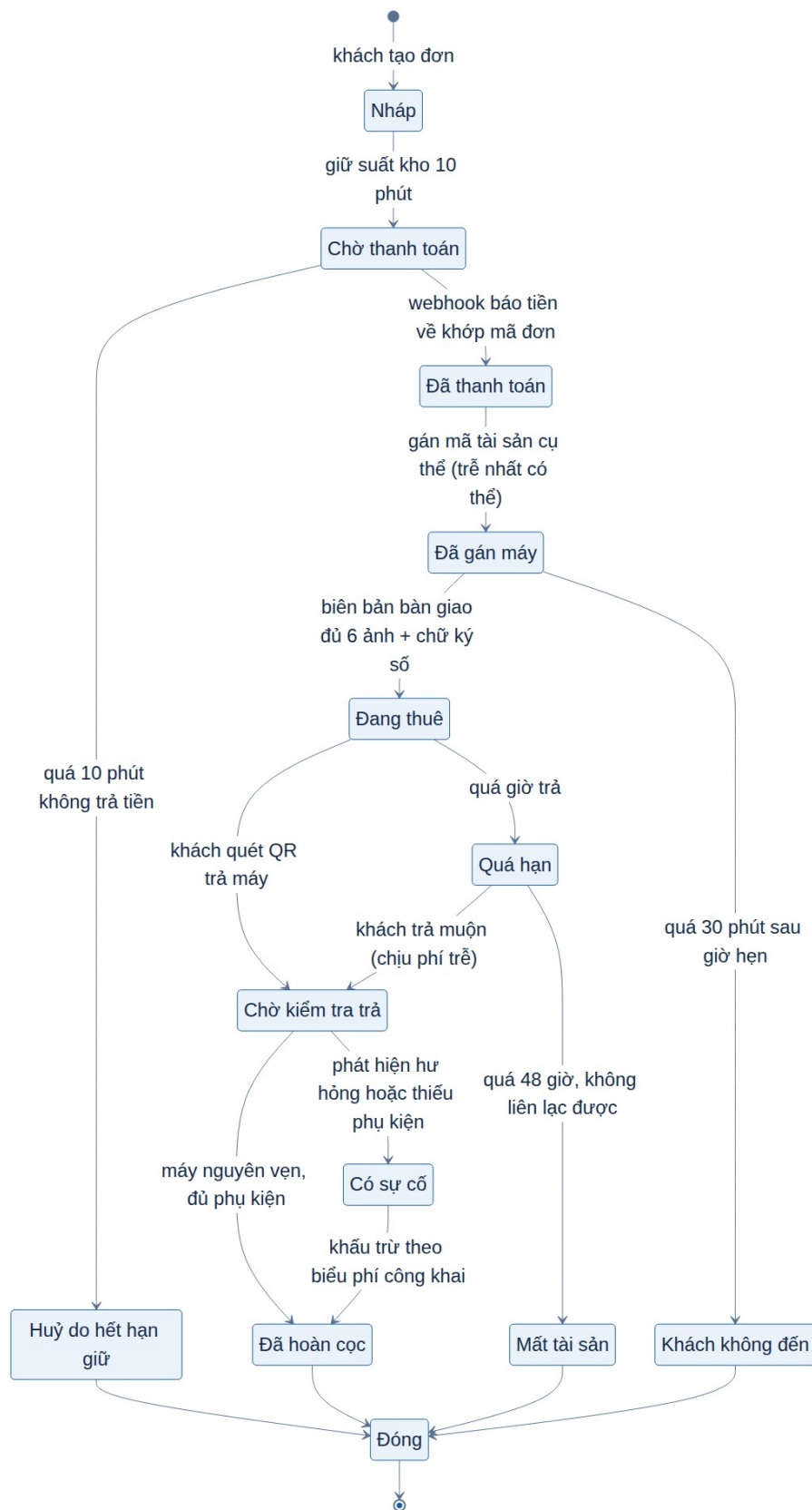
Hình 5. Máy trạng thái của một đơn thuê, mười ba trạng thái với các nhánh quá hạn, sự cố và mất tài sản.
