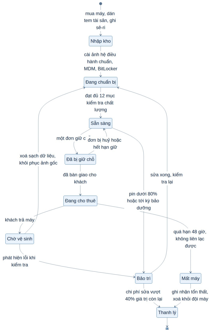
Hình 3. Vòng đời một thiết bị, từ nhập kho qua các chu kỳ cho thuê và bảo trì tới quyết định thanh lý.
