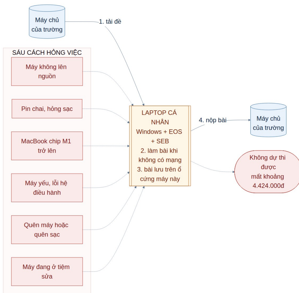
Hình 1. Luồng dữ liệu của một ca thi EOS và sáu cách chiếc laptop cá nhân có thể làm hỏng cả buổi thi.
