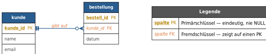
ER-Diagramm: ein kleines Beispiel und die Notation
