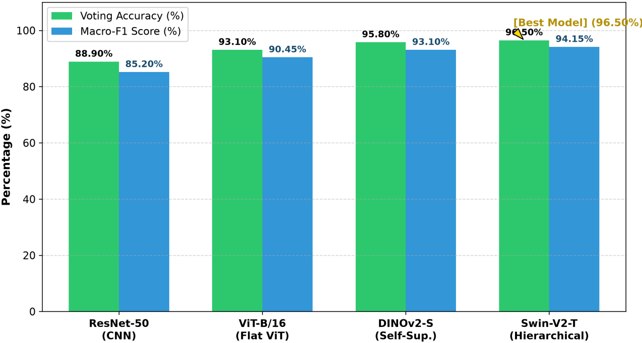
Hình 2: Biểu đồ so sánh trực quan hiệu năng giữa 4 mô hình (Voting Accuracy & Macro-F1) trên tập dữ liệu đợt 3.
