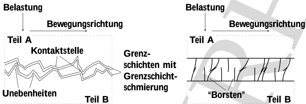
(a) Mikroskopische Ansicht eines Kontaktbereichs mit (Oberflächen-)Unebenheiten und Kontaktstellen (Darstellung basiert auf Abb. 4 in [6]).
