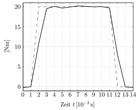
(a) Momentenerzeugung mit Verzögerung von \approx 2 \cdot 10^{-3} [s]: --- u(\cdot) = m_{M,\text{ref}}(\cdot) und — m_M(\cdot) = \text{sat}_{\hat{u}_A}(u(\cdot) + u_A(\cdot)) .
