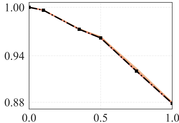
CVaR
