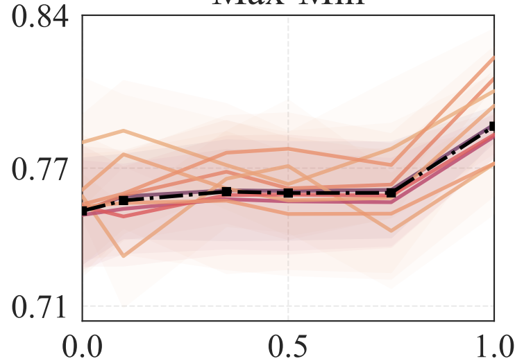
Max-Min
