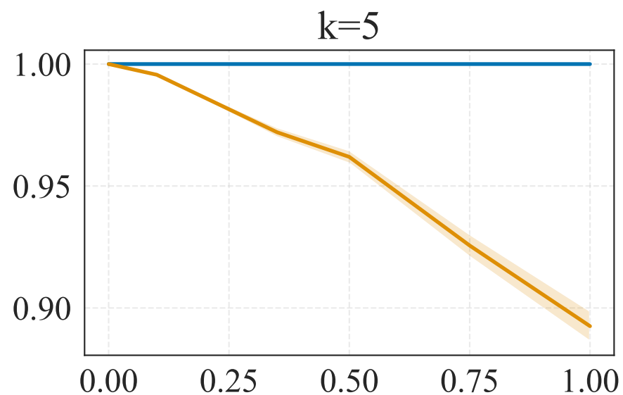
MovieLens
